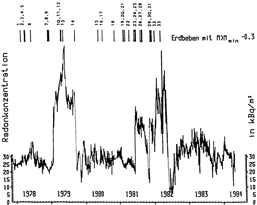
Abb. 1: Der Radongehalt der Freibadquelle sowie alle Erdbeben, die die Relation M \geq 2,4 \cdot \lg(d) - 0,43 - 0,3 erfüllen.
