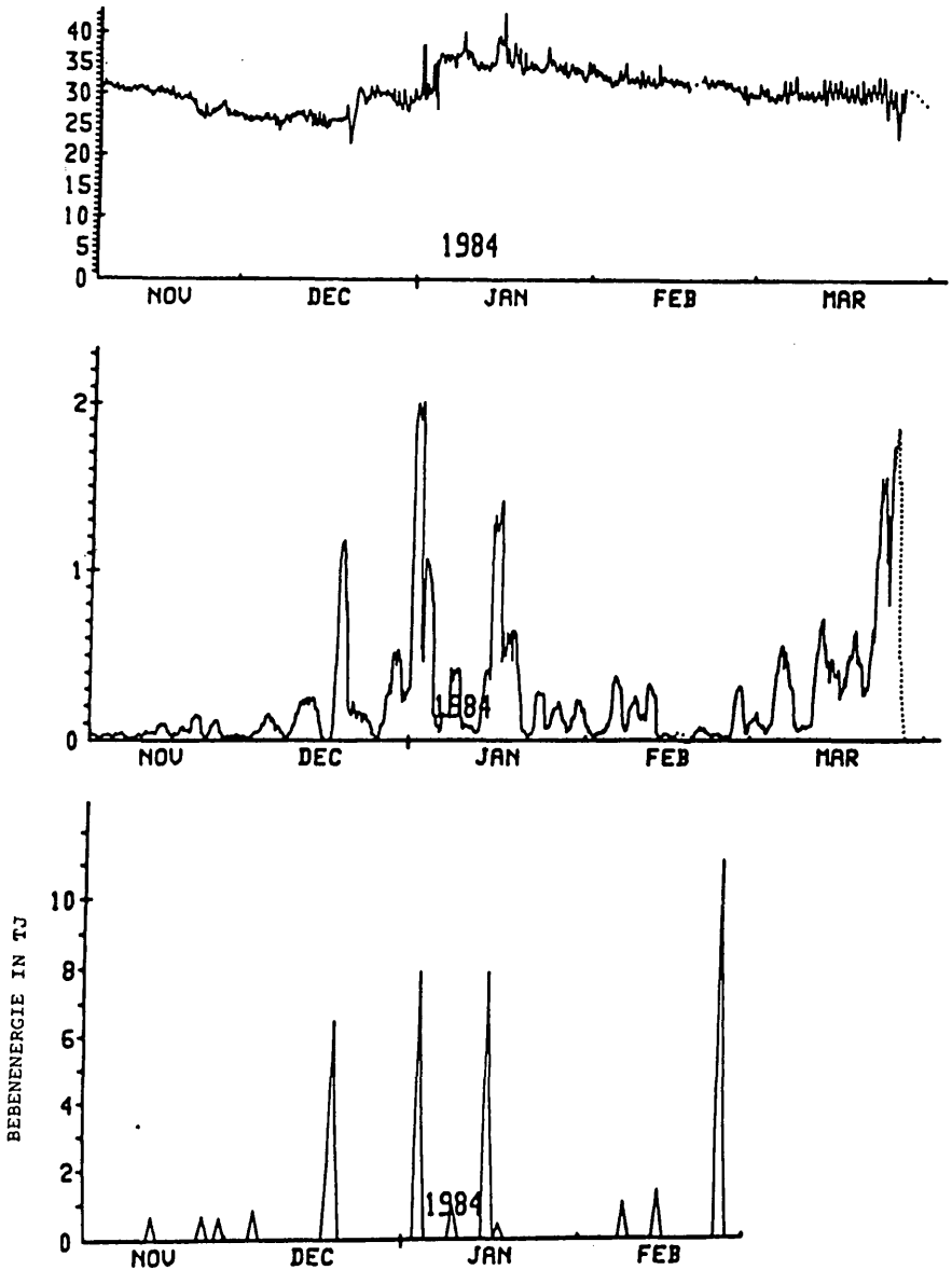
Abb. 6: Bebenenergie, Radonfluktuationsfunktion und Radonkonzentration, Winter 1983/84.
