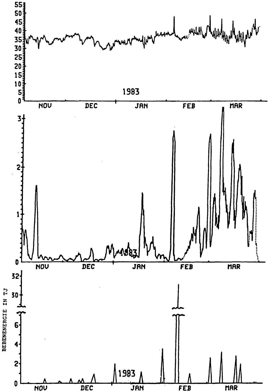
Abb. 5: Bebenenergie, Radonfluktuationsfunktion und Radonkonzentration, Winter 1982/83.
