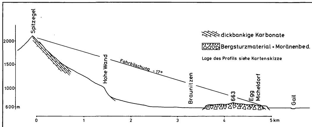
Abb. 5: Profil entlang des Stromstriches des Bergsturzes.
