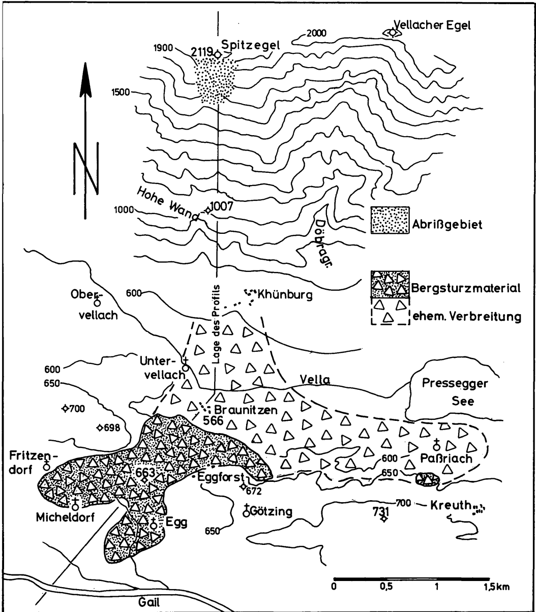
Abb. 2: Kartenskizze des Bergsturzgebietes.
