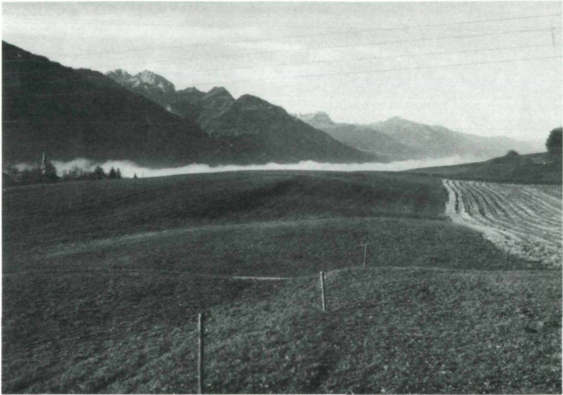
Abb. 3: Glazial überformte Oberfläche des Bergsturzmateriels. Links im Bildmittelfund der Kirchturm von Egg.
