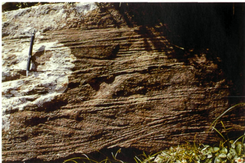
Abb. 4: Feinkörniger Sandstein mit Hummocky-Schrägschichtung, Kronalpe-Ostseite.
