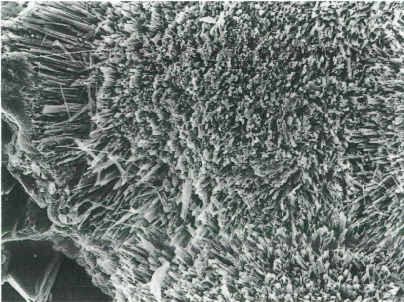
Abb. 3: Radialstrahlige angeordnete Kristalle eines mit Eosphorit verwandten Ca-Al-Mn-Fe-Phosphates, Weinebene, Koralpe. Bildbreite 0,25 mm (REM-Aufnahme: Zentrum für Elektronenmikroskopie Graz)
