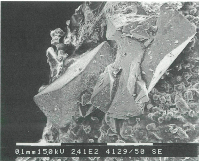
Abb. 9: Verzernte Jarositskristalle, Oberhaag. Bildbreite 0,5 mm (REM-Aufnahme: Zentrum für Elektronenmikroskopie Graz)
