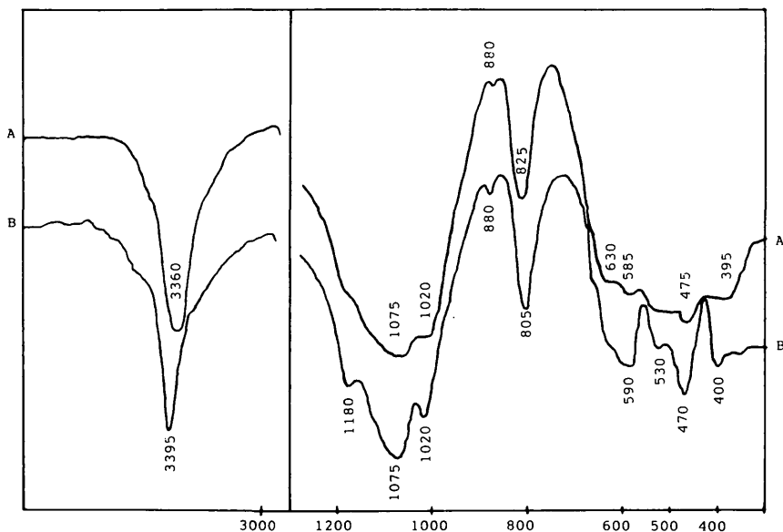
Abb. 1: IR-Spektren von Amblygonit, Montebrasit (A) und von Montebrasit, Wein-ebene, Koralpe (B), (KBr-Preßlinge)
