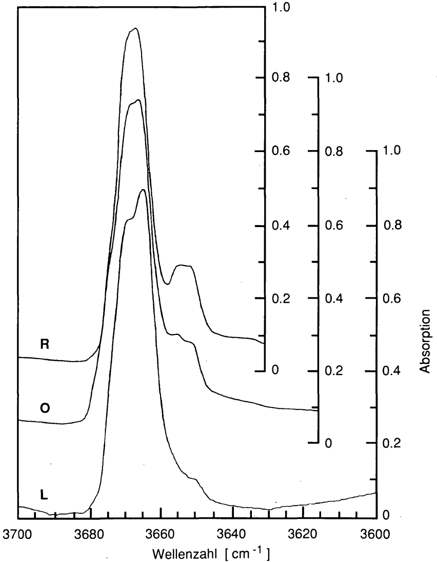
Abb. 1: Infrarotspektren von den Anthophylliten/Roßalm (R), Ochsenkogel (O) (WALITZI et al., 1989) und St. Leonhard (L).
