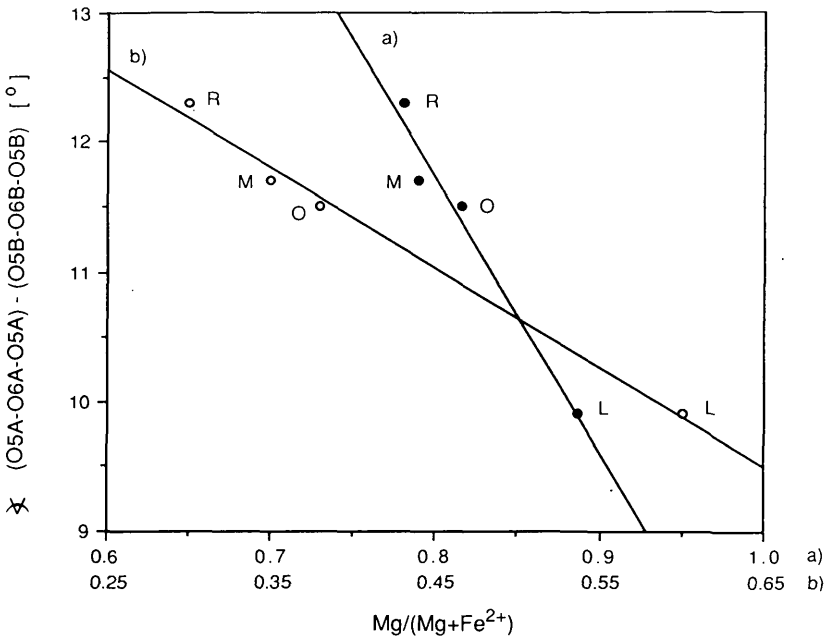
Abb. 3: Für die Anthophyllite/St. Leonhard (L), Montana (M) (FINGER, 1970), Ochsenkogel (O) (WALITZI et al., 1989) und Roßalm (R) ist die Differenz der O5-O6-O5-Winkel in der A- und B-Tetraederkette gegen das Mg/(Mg + Fe^{2+}) -Verhältnis a) in M1-M4 (volle Kreise) und b) in M4 (leere Kreise) aufgetragen.
