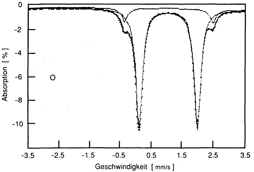
Abb. 2: Mößbauerspektren von Anthophyllit/Roßalm (R) und von Anthophyllit/Ochsenkogel (O) (WALITZI et al., 1989).
