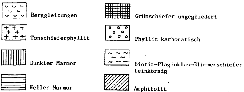
Abb. 1: Geologische Karte des Trixener Tales (vereinfacht nach der „Geologischen Karte der Saualpe-Süd“, GEOLBA Wien, 1978).
