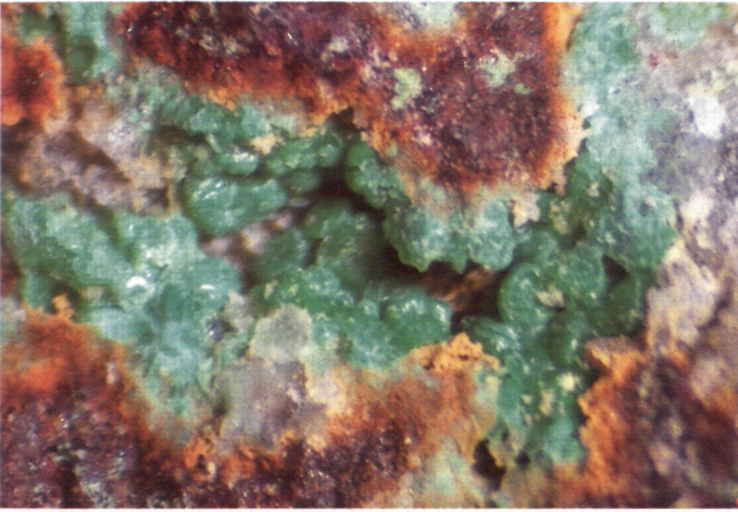
Abb. 3: Parnait in kugeligen Aggregaten auf Quarz (Ausmaß 2 mm); Rijavitzza-Graben. Foto und Sammlung: M. PUTTNER.
