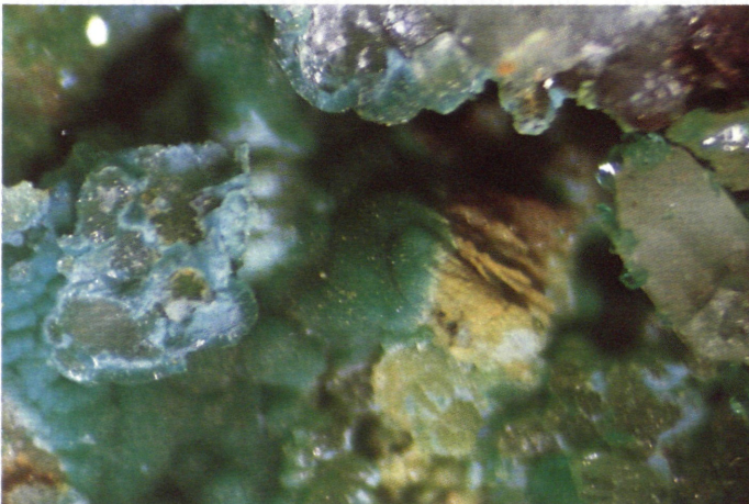
Abb. 4: Paragenese aus überwiegend Parnait, verwachsen mit hellblauem Clarait sowie idiomorph entwickelten Chalkophyllit-Tafeln auf einem Bergkristall (Vergrößerung 30fach); Rijavitzza-Graben. Foto und Sammlung: M. PUTTNER.
