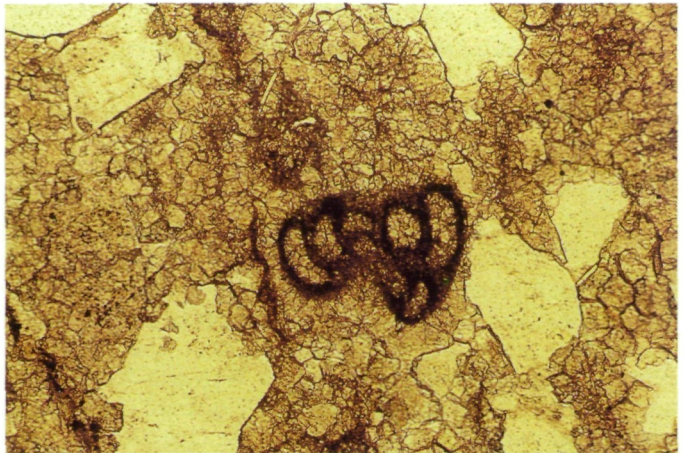
Abb. 27: Mikroskopische Dünnschliffaufnahme eines feinkörnigen Sandsteins aus den Werfener Schichten bei Untermitterdorf, bestehend aus karbonatisch zementierten Quarz- und Feldspatkörnern. In der Bildmitte ist eine Foraminifere erkennbar. Bildausschnitt ca. 3 x 5 mm.
