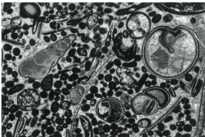
Abb. 4: Mikroskopische Dünnschliffaufnahme eines Gastropodenoolithes aus den südalpinen Werfener Schichten im Ardeschitzagraben südlich von Rosenbach, bestehend aus rundlichen, dunklen Ooiden und Schalenresten von überwiegend Gastropoden. Bildausschnitt ca. 10 x 16 mm.
