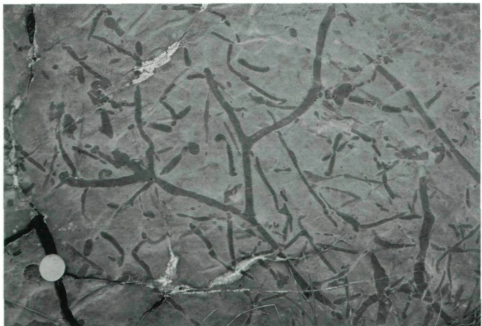
Abb. 19: Grauer, mikritischer Wurstelkalk mit schön erhaltenen Lebensspuren ( Thalassinoides ), aufgeschossen am Staff, westlich des Gipfels.
