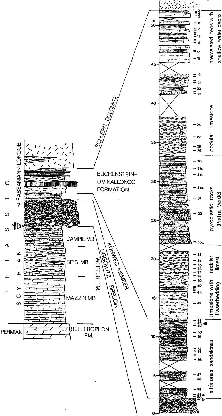
Abb. 15: Profil durch die südälpine Triasabfolge im Gartnerkofelgebiet, Karnische Alpen (aus KOZUR et al., 1994, Abb. 2).
