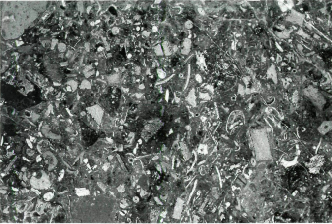
Abb. 6: Mikroskopische Dünnschliffaufnahme eines Rotkalke der Loibl-Formation. Der Kalk besteht aus zahlreichen Bruchstücken und verschiedenen Schalenresten in einer mikritischen Grundmasse. Aufschluß an der Zelenica-Forststraße westlich des Loibltunnels, Bildausschnitt ca. 10 x 16 mm.
