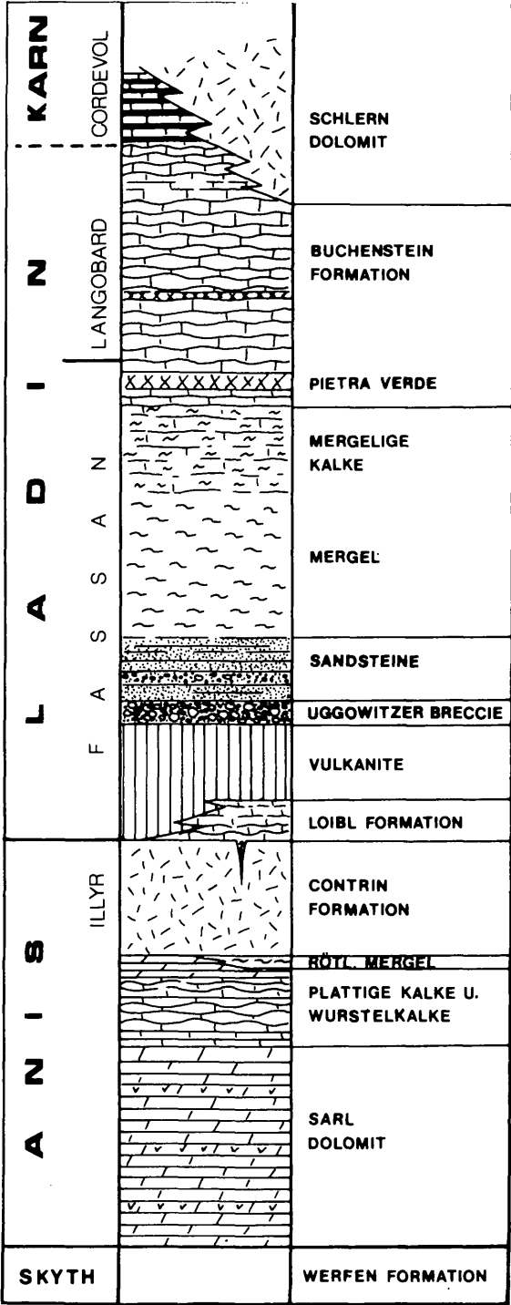
Abb. 5: Übersichtsprofil durch die südalpine Mitteltrias (Anis – Ladin) der zentralen Karawanken zwischen dem Bärntal und der Koschuta.
