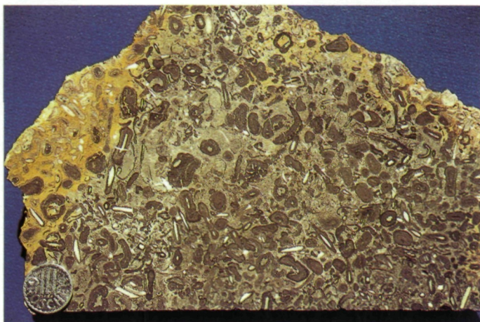
Abb. 24: Onkolith (Anschnitt) aus den Raibler Schichten, die entlang des Forstweges von Rubland in den Kreuzengraben aufgeschlossen sind.
