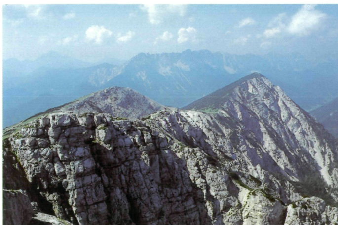
Abb. 26: Das Gipfelmassiv des Hochobirs besteht aus dickbankigem Wettersteinkalk der Lagunenfazies (Vordergrund). Blick vom Gipfel des Hochobirs nach Südwesten, im Hintergrund die Koschuta.
