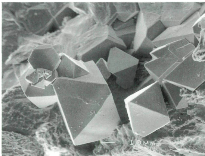
Abb. 2: Senarmontit bildet in Kavernen des Antimonerzes von Leßnig nicht selten dichte Rasen okta- edrischer Kriställ- chen. REM-Aufnah- me. Bildbreite: ca. 0,15 mm.
