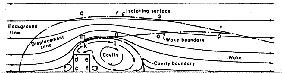
Abb.5: Strömungsverhalten an einem dreidimensionalen Hinderniss. (aus HALITSKY 1968).
