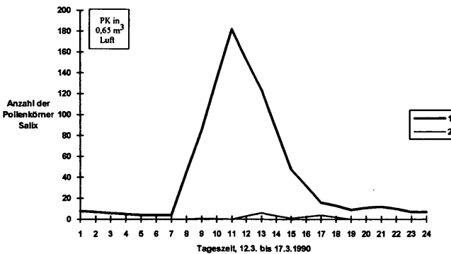
Abb. 22: Summenkurven der Tagesverteilungen des Salix -Pollenfluges vom 12. 3. bis 17. 3. 1990. 1: Salix -Pollenflug beim Standort 1. 2: Salix -Pollenflug im Stadtgebiet von Klagenfurt.
