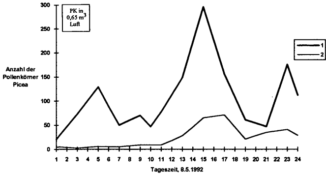
Abb. 28: Tagesverlauf des Picea -Pollenfluges am 8. 5. 1992. 1: Picea -Pollenflug beim Standort 19. 2: Picea -Pollenflug im Stadtgebiet von Klagenfurt.
