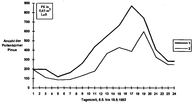
Abb. 32: Summenkurven der Tagesverteilungen des Pinus -Pollenfluges vom 6. 5. bis 18. 5. 1992. 1: Pinus -Pollenflug beim Standort 19. 2: Pinus -Pollenflug im Stadtgebiet von Klagenfurt.
