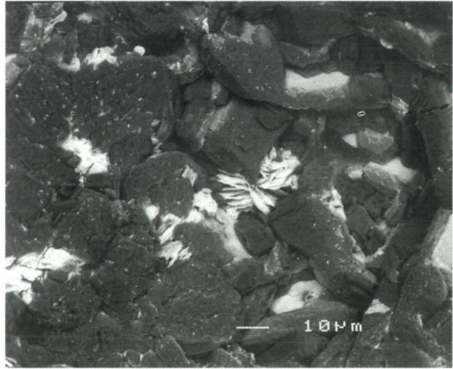
Abb. 10: Aggregat dünn- tafeliger Schröckingeritkristalle (Bildmitte, weiß) in Gips (dunkelgrau) von der Kölnbreinsperre im Maltatal, Kärnten. Bildbreite ca. 0,15 mm. REM-Aufnahme (BSE-Modus): NHM Wien.
