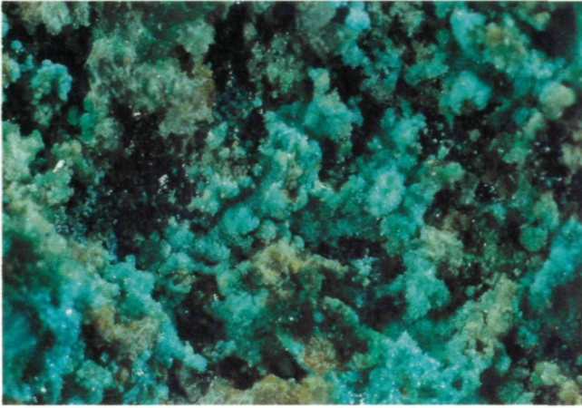
Abb. 4: Feinste schuppig-blättrige Aggregate von Klinotiroilit auf Malachit vom Rijavitzagraben. Bildbreite 4mm. Foto: H. W. Graf.
