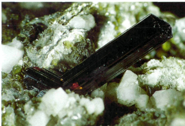
Abb. 21: Typischer Rutil-„Kniezwillinger“ von Grieswies-Mähder in der Rauris, Salzburg. Bildbreite 1 cm. Sammlung und Foto: NHM Wien.
