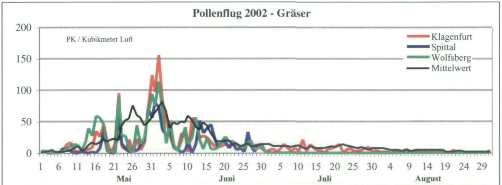
Abb. 8: Vergleichskurven des Pollenfluges der Gräser (Poaceae) im Jahr 2002
