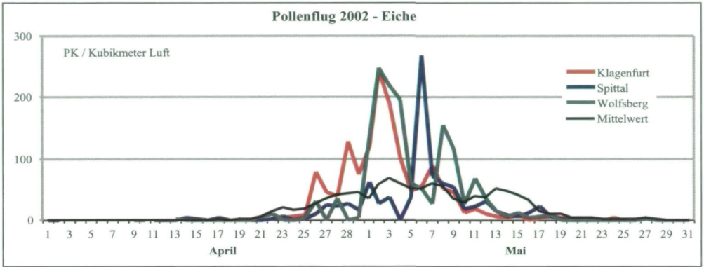
Abb. 7: Vergleichskurven des Pollenfluges der Eiche ( Quercus sp.) im Jahr 2002
