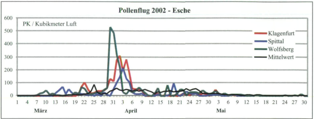
Abb. 5: Vergleichskurven des Pollenfluges der Esche ( Fraxinus excelsior ) im Jahr 2002
