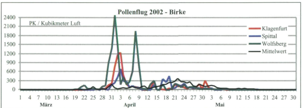
Abb. 6: Vergleichskurven des Pollenfluges der Birke ( Betula pendula ) im Jahr 2002
