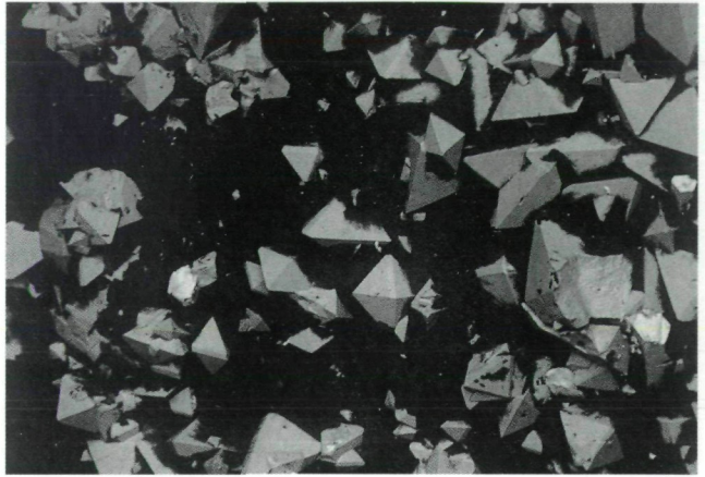
Abb. 11: Nur bis 0,1 mm große, aber modellar- tig ausgebildete Descloizite vom alten Bergbau Fuchsriegel bei Schwarzenbach im Pielachtal, Niederösterreich. REM-Aufnahme (BSE-Modus); NHM Wien, F. Brandstätter.
