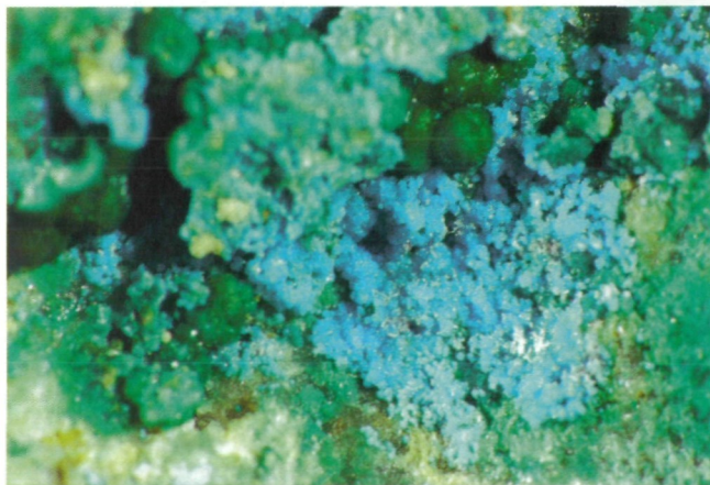
Abb. 3: Strashimirit wird oft von himmelblauem Richelsdorffit überkrustet. Rellstal im Montafon, Vorarlberg. Bildbreite 4 mm. Foto: G. Niedermayr.
