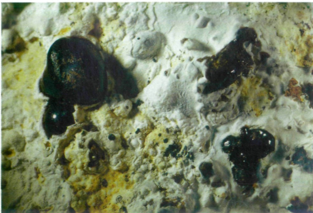
Abb. 7: Nierig-traubige Krusten von dunkel bräunlichrotem Hydronium-Jarosit (aus dem ehemaligen Graphitabbau am Weinberg bei Amstall, Nieder- österreich) werden von einem feinst- kristallinen Belag aus Gips, Illit und Quarz überwachsen. Bildbreite 2 cm. Sammlung: Erwin Löffler, Emmers- dorf/Donau. Foto: G. Niedermayr.
