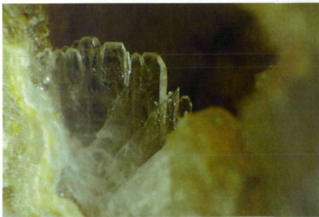
Abb. 14: Baryt-Aggregat in einem Hohlraum im Leithakalk S Sommerein, Niederösterreich. Bildbreite 5 mm. Foto: G. Niedermayr.
