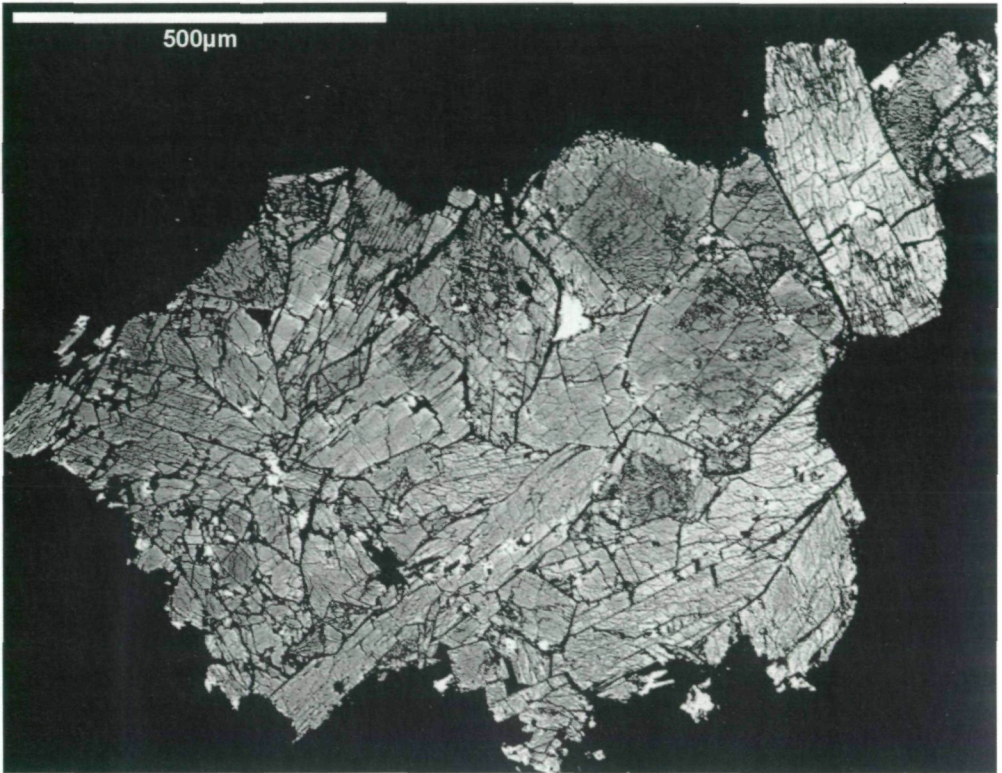
Abb. 2: Polierter Anschliff von Laumontit, Wurten. Elektronenmikroskopische Abbildung rückgestreuter Elektronen (BSE).
