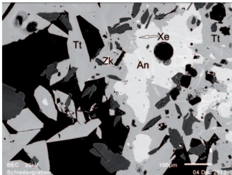
Abb. 27: REM-Aufnahme eines Anschliffes von Titanit der jüngeren Generation (Tt) mit Einschlüssen von Anatas (An), Zirkon (Zk) und Xenotim (Xe), Schiedergraben im Felbertal, Salzburg. Balkenmaßstab 0,1 mm. Das kreisrunde Loch wurde durch eine Laser-Ablations-Analyse verursacht. Foto: H.-P. Bojar
