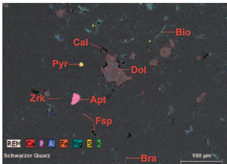
Abb. 31: Elementverteilung eines Axialschnitts durch einen schwarzen Bergkristall vom Gipfel des Weisseck, Salzburg. Deutlich zu erkennen ist die große Anzahl von Einschlüssen (v. a. Biotit), die farbgebend sein dürften. Apt: Fluorapatit, Bio: Biotit, Bra: Brannerit, Cal: Calcit, Dol: Dolomit, Fsp: Feldspat, Pyr: Pyrit, Zrk: Zirkon. Hypermap: C. Steinwender
