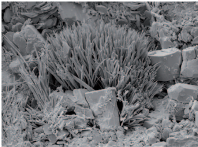
Abb. 35: Etwa 30 µm großer tafeliger Anatas- Kristall, umsäumt von feinnadeligem Malachit aus dem Gipsbruch Pfen- nigbach, Nieder- österreich. REM-Foto (BSE- Modus); Ch. Auer
