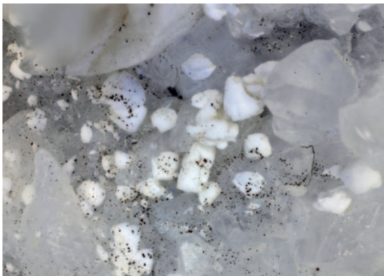
Abb. 14: Baryt als milchig-weiße, gerundet blockige Kriställchen, von winzigen Pyriten überstäubt und auf Calcitkristallen sitzend. Steinbruch Rhomberg bei Hohenems, Vorarlberg. Bildbreite 7 mm. Sammlung: NHM Wien. Foto: H. Schillhammer
