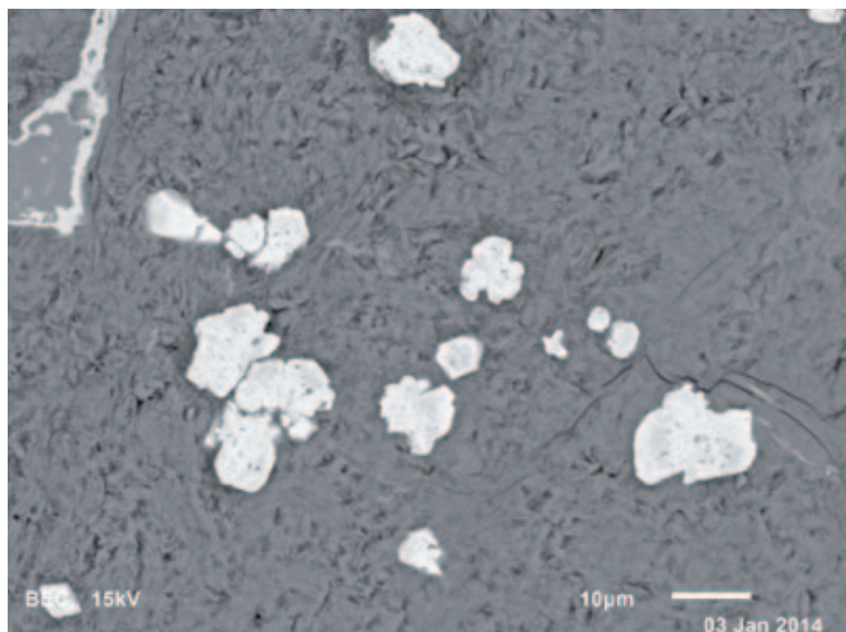
Abb. 19: Sr-reicher Florencit-(Ce) bildet winzige, in feinblättrigen Muskovit eingewachsene Kristall- aggregate in einem mit Sulfiden leicht vererzten Magnesit- reichem Anschliff vom unteren Rellstal im Montafon, Vorarl- berg. Sammlung: NHM Wien. REM-Foto (BSE- Modus) U. Kolitsch
