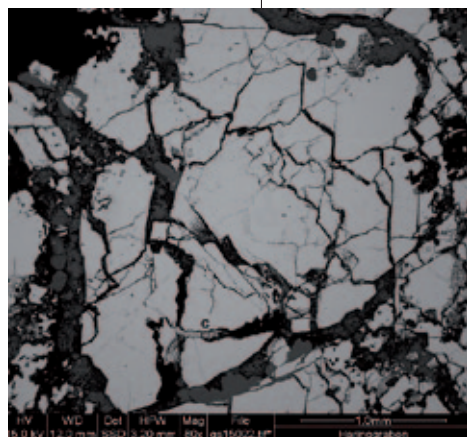
Abb. 43: Coelestin als Rissfüllung in Sphalerit mit Calcit und Gips vom Haringgraben, Tragöß-Oberort, Steiermark. REM-Foto (BSE-Modus): Zentrum für Elektronenmikroskopie Graz.
