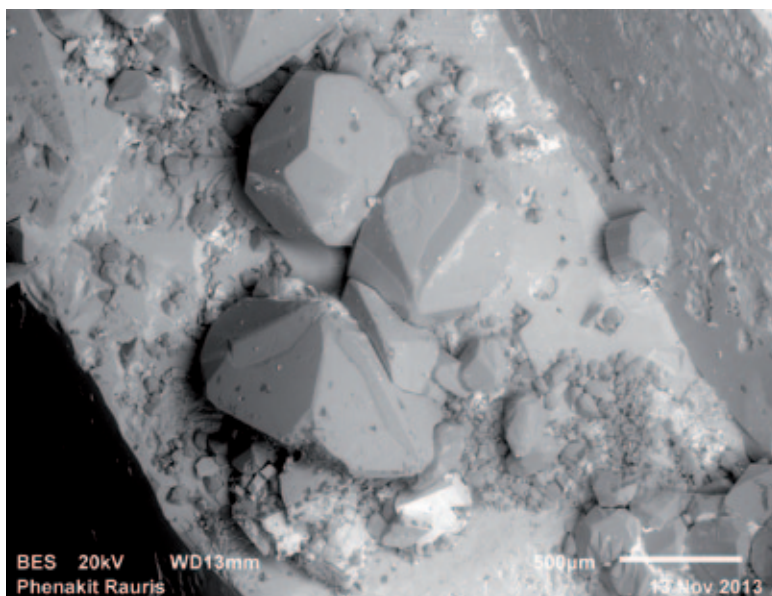
Abb. 28: REM-Aufnahme von Phenakit mit kurz- prismatischem bis linsenförmigem Ha- bitus und typischer Verwilligung („Fräserkopf“) auf Quarz, Erfurter- steig, Grießwies- Schafkar, Rauris, Salzburg; Balken- maßstab 0,5 mm.
