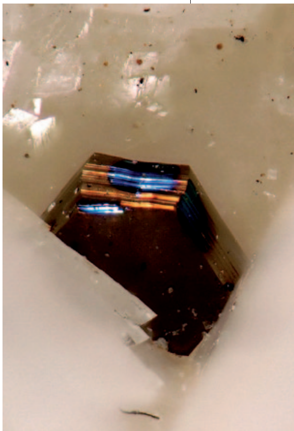
Abb. 29: Pyrrhotinkristall auf Dolomit aus dem Schönberg-Tunnel bei Schwarzach- St. Veit, Salzburg. Bildbreite 1,8 mm. Sammlung: Universalmuseum Joanneum. Foto: W. Trattner
