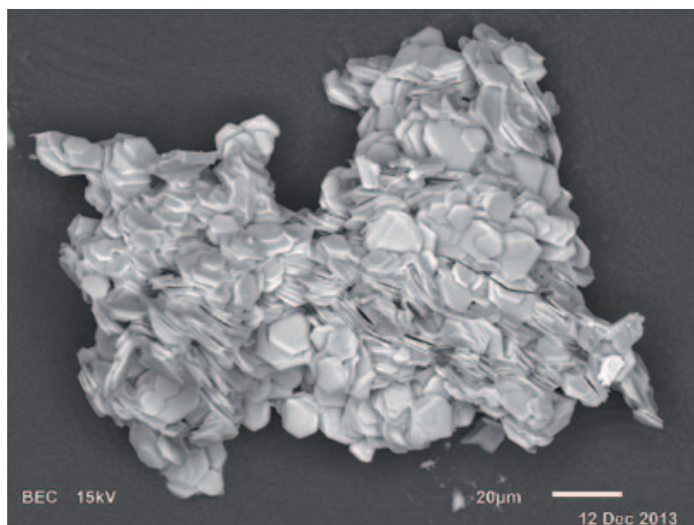
Abb. 45: Der hellgelbbraune bis blassrötlichbraune Slavíkit vom Prenterwinkelgraben, Steiermark, bildet typische sechsseitige Täfelchen; Sammlung: H. Schabereiter. REM-Foto (BSE-Modus); U. Kolitsch
