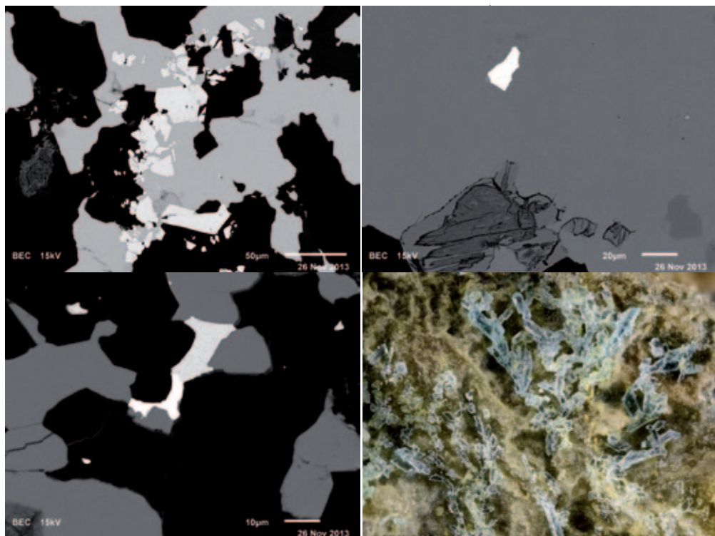
Abb. 22: Typische Beispiele der artenreichen Mineralisation vom alten Bergbau am Nordhang des Valschavielkopfes bzw. Eisernen Tors, Alpe Fresch im Silbertal, Montafon, Vorarlberg. Fotos 21a–21c, Sammlung: NHM Wien. REM-Foto (BSE-Modus): U. Kolitsch
