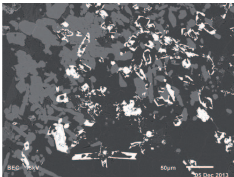
Abb. 20: Prismatische Fluorapatitkristalle neben Arsenopyrit- hohlkristallen. Man- che der Arsenopy- rite enthalten Kerne aus Tetraedrit, die meisten jedoch Mg-haltigen Siderit. Erzanschliff von der Knappagruaba, Bartholomäberg im Montafon, Vorarl- berg; Sammlung: NHM Wien. REM-Foto (BSE-Modus): U. Kolitsch
