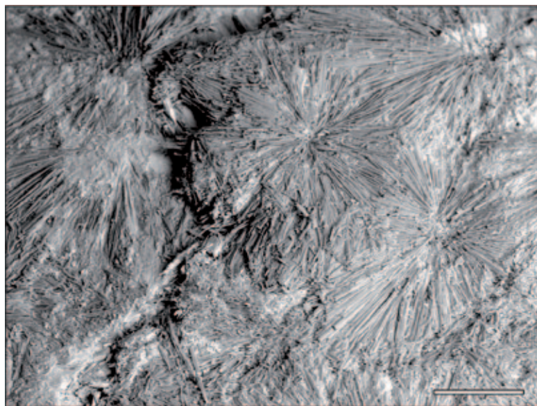
Abb. 3: REM-Aufnahme von radialstrahlig angeordneten Dawsonit- Kristallen auf einer Kluftfläche des Granits von Eisen- kappel, Ebriacher Sauerbrunn bei Bad Eisenkappel, Kärnten. Balken- maßstab 0,2 mm. Foto: H.-P. Bojar
