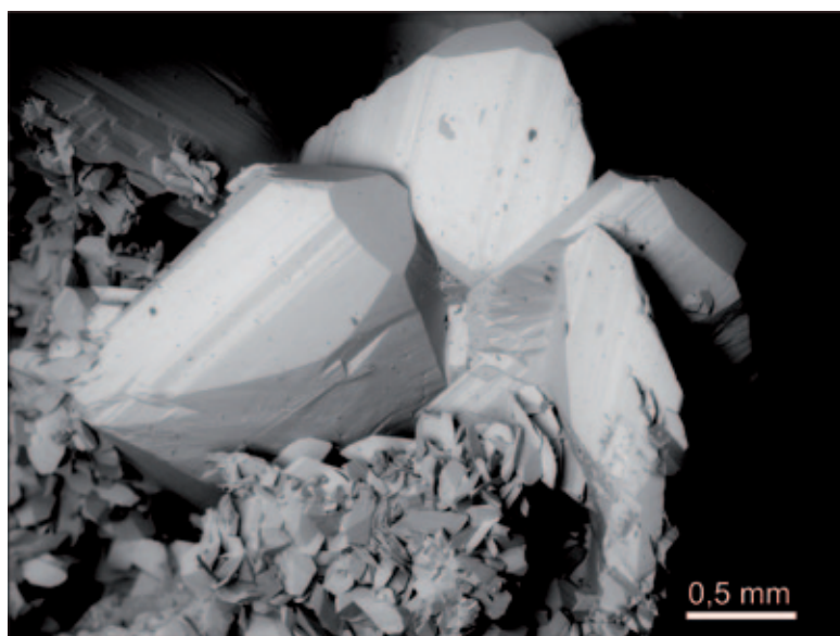
Abb. 26: REM-Aufnahme von verzwillingten Tita- nitkristallen (große Kristalle), die von Titanit der jüngeren Generation über- wachsen werden, Schiedergraben im Felbertal, Salzburg. Balkenmaßstab 0,5 mm. Foto: H.-P. Bojar
