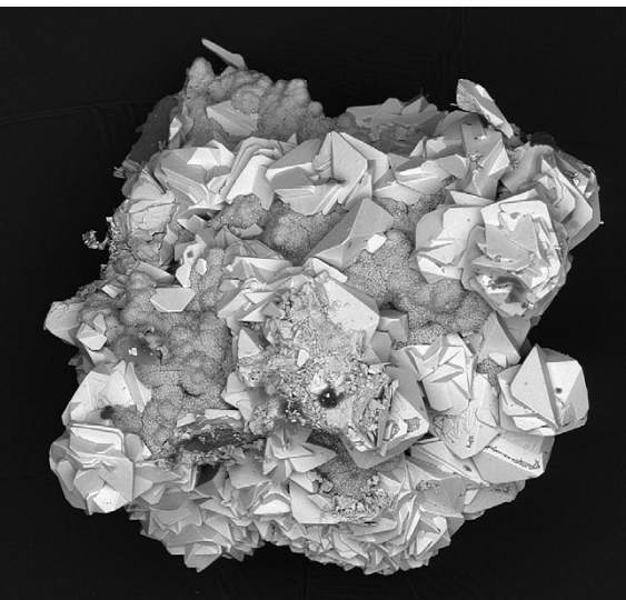
Abb. 5: Segnititkristalle von Guginock bei Lind im Drautal, Kärnten; Bildbreite 0,65 mm. REM-Foto (BSE-Modus): C. Auer
