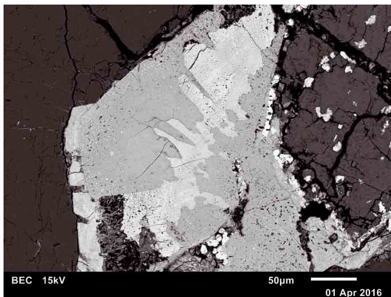
Abb. 23: Eine komplexe Paragenese von akzessorischen Pegmatitmineralien vom Blocherleiten-graben im Mieslingtal bei Spitz (Anschliff): kleine Cheralith-Körner (hell) sitzen randlich an einer dendritenartigen Verwachsung von Xenotim-(Y) (hellgrau, leicht zoniert) und Zirkon (grau, porös). Links unten ein Anwachsraum eines Y-, P- und weitere Fremdelemente enthaltenden, chemisch inhomogenen Zirkons. Rechts oben eine nicht identifizierte Fe-Al-Si-O-Phase (dunkel), links Quarz (sehr dunkel). Sammlung: NHM Wien und REM-Foto (BSE-Modus): U. Kolitsch
