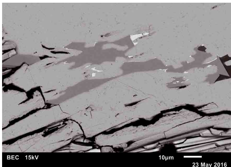
Abb. 11: Xenomorpher Ull- mannit (grau), verwachsen mit wenig Galenit (weiß), beide ein- geschlossen in Jamesonit (hell- grau). „Jamesonit“- Stufe von „Wiltau, Tirol“ (Inventar- nummer A. a. 7863), Sammlung: NHM Wien und REM-Foto (BSE- Modus): U. Kolitsch
