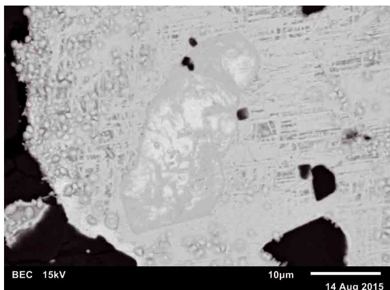
Abb. 29: Marrit (hell) als xenomorphe, reliktitische Körner innerhalb eines Proustit-Korns (mittelgrau), das wiederum in Billingsleyit (hellgrau, z. T. mit Gittertextur) eingeschlossen ist. Der Billingsleyit zeigt körnige Akanthit-Ausblühhungen. Anschliff einer Erzprobe von der Halde des 1. Zubautollens der Grube Anna, Annaberg, Niederösterreich. Sammlung: NHM Wien und REM-Foto (BSE-Modus): U. Kolitsch
