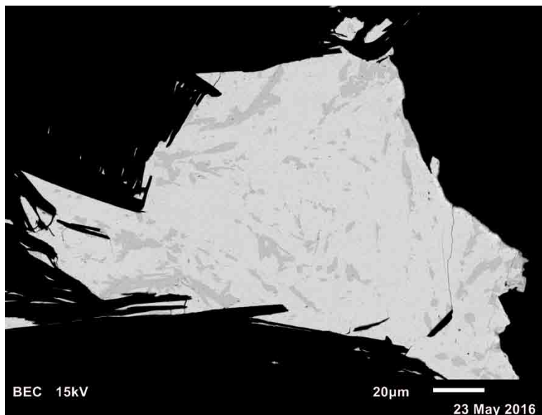
Abb. 10: Boulangerit (hell), darin eingeschlos- sen etwas Jameso- nit (hellgrau), in Quarz-Muskovit- Matrix (schwarz). „Jamesonit“-Stufe von „Wiltau, Tirol“ (Inventarnummer A.a. 7863). Sammlung: NHM Wien und REM-Foto (BSE- Modus): U. Kolitsch
