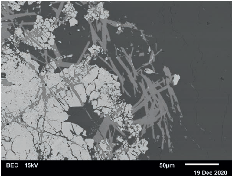
Abb. 29: Coombsit als miteinander verwachsene, lattige Kristalle (grau) in Albit (dunkel). Links Aggregate von körnigem Braunit (hellgrau) mit schmalen Rhodochrosit-Rissfüllungen (grau). Sammlung: NHM Wien (MPA-Inventar-Nr. O 2105). REM-Foto (BSE-Modus): U. Kolitsch
