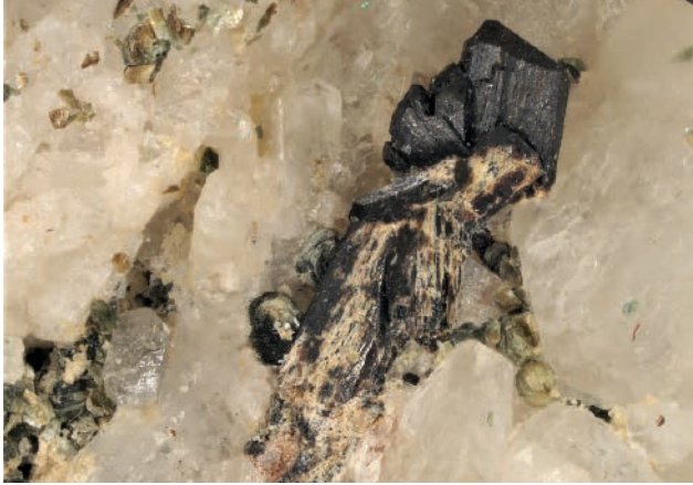
Abb. 8: Gruppe schwarzer Polykras-(Y)-Kristalle auf Albit und Adular mit Chlorit aus einer alpinen Kluft östlich der Gamolnigspitze, Reißeckgruppe, Kärnten. Bildbreite 6 mm. Foto: H.-P. Bojar
