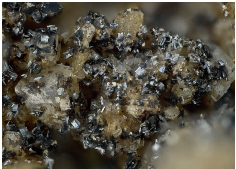
Abb. 17: Schwarze, rechtwinklig begrenzte Pyrolusit-Täfelchen auf blassbräunlichen bis farblosen, leicht gerundeten Dolomit-Rhomboedern. Inaktiver Magnesitbergbau Bürglkopf südwestlich von Hochfilzen, Tirol. Bildbreite: 3,5 mm. Sammlung: NHM Wien (MPA-Inventar-Nr. O 2111). Foto: H. Schillhammer
