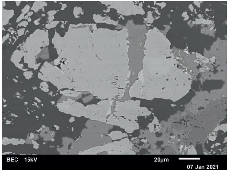
Abb. 32: Die größten im untersuchten Anschliff gefundenen Körner des unbenannten Epidotgruppen-Minerals \text{CaSr}(\text{Fe}^{3+}\text{AlMn}^{3+}) (\text{Si}_2\text{O}_7)(\text{SiO}_4)\text{O}(\text{OH}) (hellgrau; die helleren schmalen Randsäume sind angereichert an Pb und Mn), durch- brochen von einer Rhodochrositader (dunkelgrau), einge- wachsen in Albit (dunkel). Polierter Anschliff von der Fuchsalm, Radstädter Tauern, Salzburg. Sammlung: NHM Wien (MPA-Inventar- Nr. O 2103). REM- Foto (BSE-Modus): U. Kolitsch
