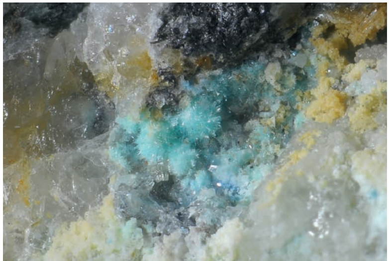
Abb. 23: Winzige himmelblaue Caledonitkristalle von den Kielbreinbauen, Radhausberg, Salz- burg. Bildbreite 2,5 mm. Foto: C. Auer
