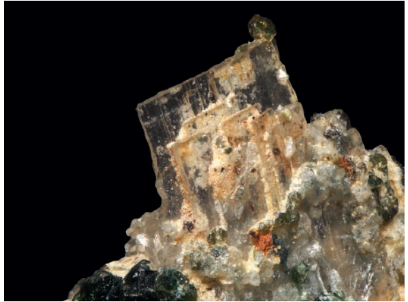
Abb. 10: Tafelige Kristalle von Bertrandit mit winzigem Titanit (Dreieck-Spiegelung) aus der alpinen Kluft östlich der Gamolnigspitze, Reißeckgruppe, Kärnten. Bildbreite 10 mm. Foto: H.-P. Bojar
