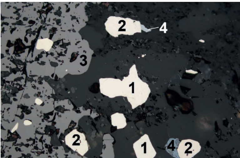
Abb. 21: Maucherit (1), Orcelit (2), Magnetit (3) und Chalkosin (4) im Nebengestein der Perowskit-Diopsid- Magnetit-Klinochlor- Calcit-Kluftminerali- sation in Serpentin- it, Brennkogel, Salzburg. Bildbreite 1 mm. Foto (Auffichtmikro- skopie): H.-P. Bojar
