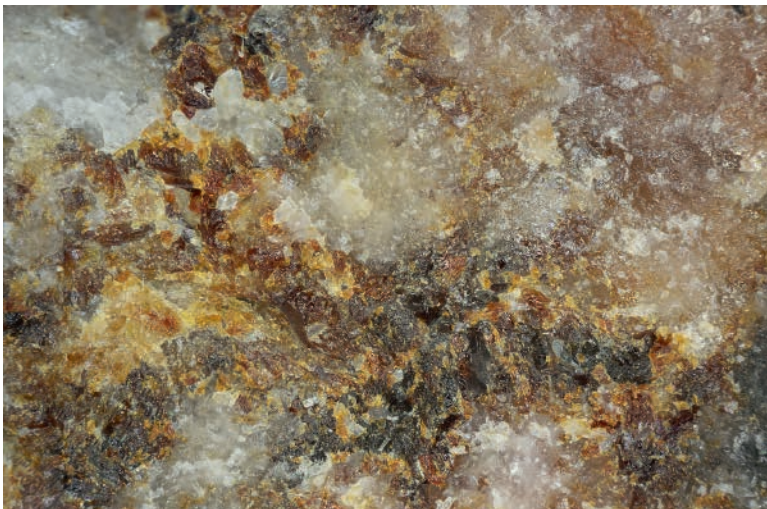
Abb. 27: Derber Arseniopleit (dunkelbraunrot) in enger Verwachsung mit etwas gelborangem Tiragalloit und blassrosa, derbem, glasigem Sarkinit (rechter Bildbereich). Fuchsalp, Radstädter Tauern, Salzburg. Bildbreite: 7 mm. Fund: T. Schachinger, Sammlung: NHM Wien (MPA-Inventar-Nr. O 2104). Foto: H. Schillhammer
