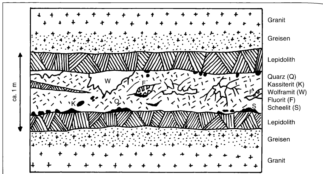
Abbildung 4. Schema des 1 m mächtigen Zinnstein-Ganges im Granit von Zinnwald im Sächsischen Erzgebirge (nach BECK 1909).
