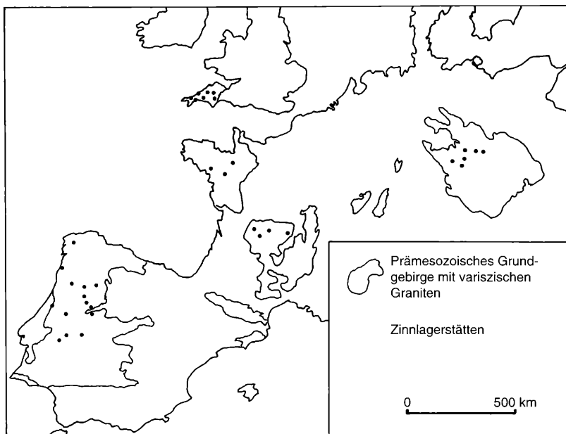
Abbildung 3. Die Verteilung der Zinn-Wolfram-Lagerstätten in den europäischen Varisziden (nach STEMPROK 1980).
