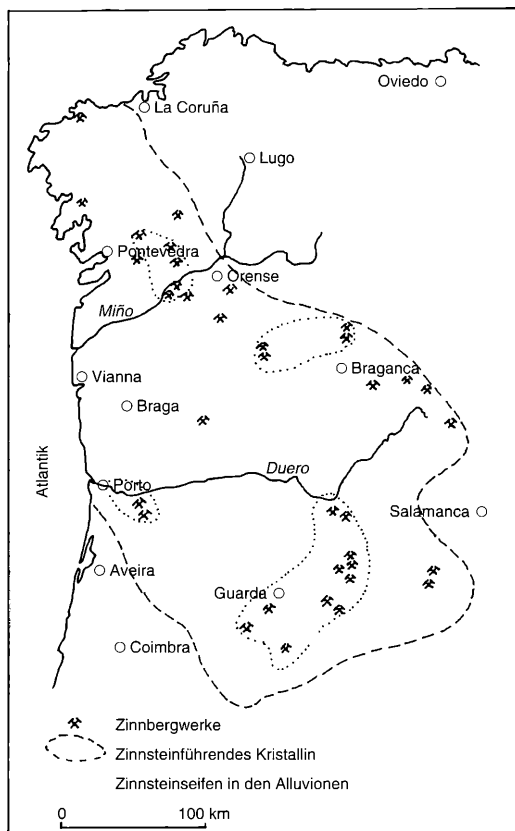
Abbildung 7 Das Zinnland in NW-Spanien und Portugal (nach QUIRING 1940)
