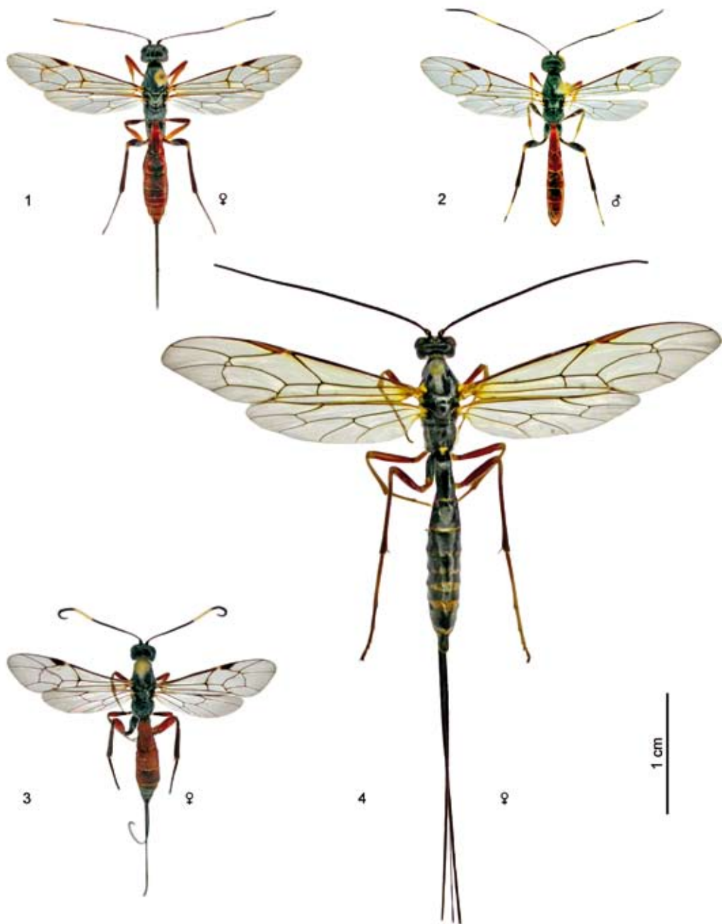
Abbildungen 1, 2. Xorides filiformis ♀, ♂ (vgl. Nr. 11 im 1. Beitrag). Die Larve entwickelt sich als Ektoparasitoid an Bockkäferlarven und vielleicht auch an Larven der Schwertwespen ( Xiphydria ). Ektoparasitoide fressen ihre Wirte von außen auf, Endoparasitoide von innen. Abbildung 3. Xorides fuligator ♀ (vgl. Nr. 12 im 1. Beitrag). Es sind noch keine Wirte bekannt. Abbildung 4. Coleocentrus excitator ♀ (vgl. Nr. 17 im 1. Beitrag). Ektoparasitoid großer Bockkäfer- und Holzwespenlarven ( Siricidae ). – Alle Fotos: J. FRICKE.
