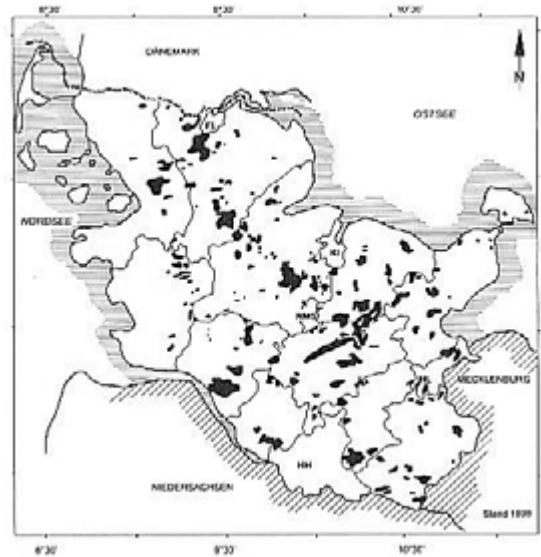
Abb.3: Vorkommen oberflächennaher, mineralischer Rohstoffe in Schleswig-Holstein ( https://www.umweltdaten.landsh.de/nuis/upool/gesamt/jahrbe97/kies/kies.htm (Zugriff 18.11.2017)). Sie bezeichnen die potentiellen Lagen für Kies-, Sand- und Tongruben. // Occurrence of near-surface, mineral raw materials in Schleswig-Holstein.
