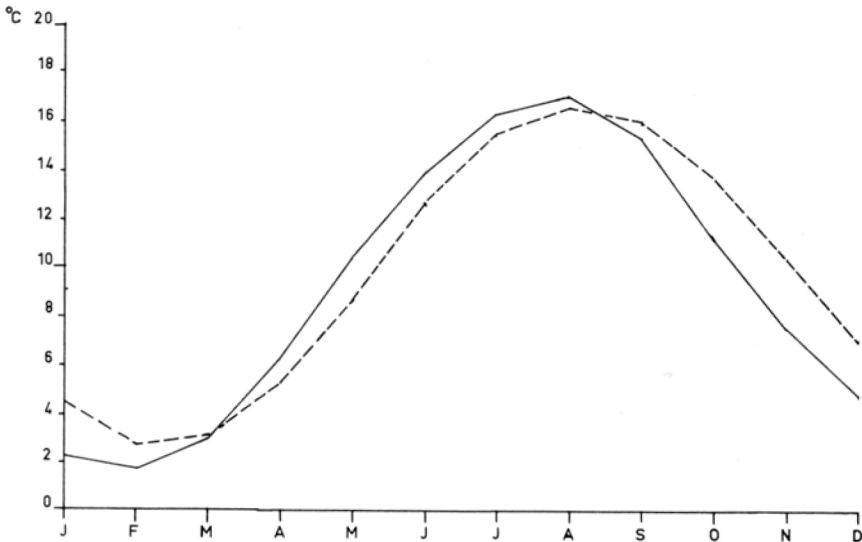
ABB. 4 20jähriges Mittel der Luft- — und Wassertemperaturen - - -
