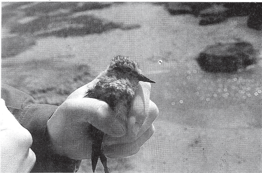
Abb. 1: Beringter nfl. Steinwälder am 30.6.1982 in Nordfriesland
