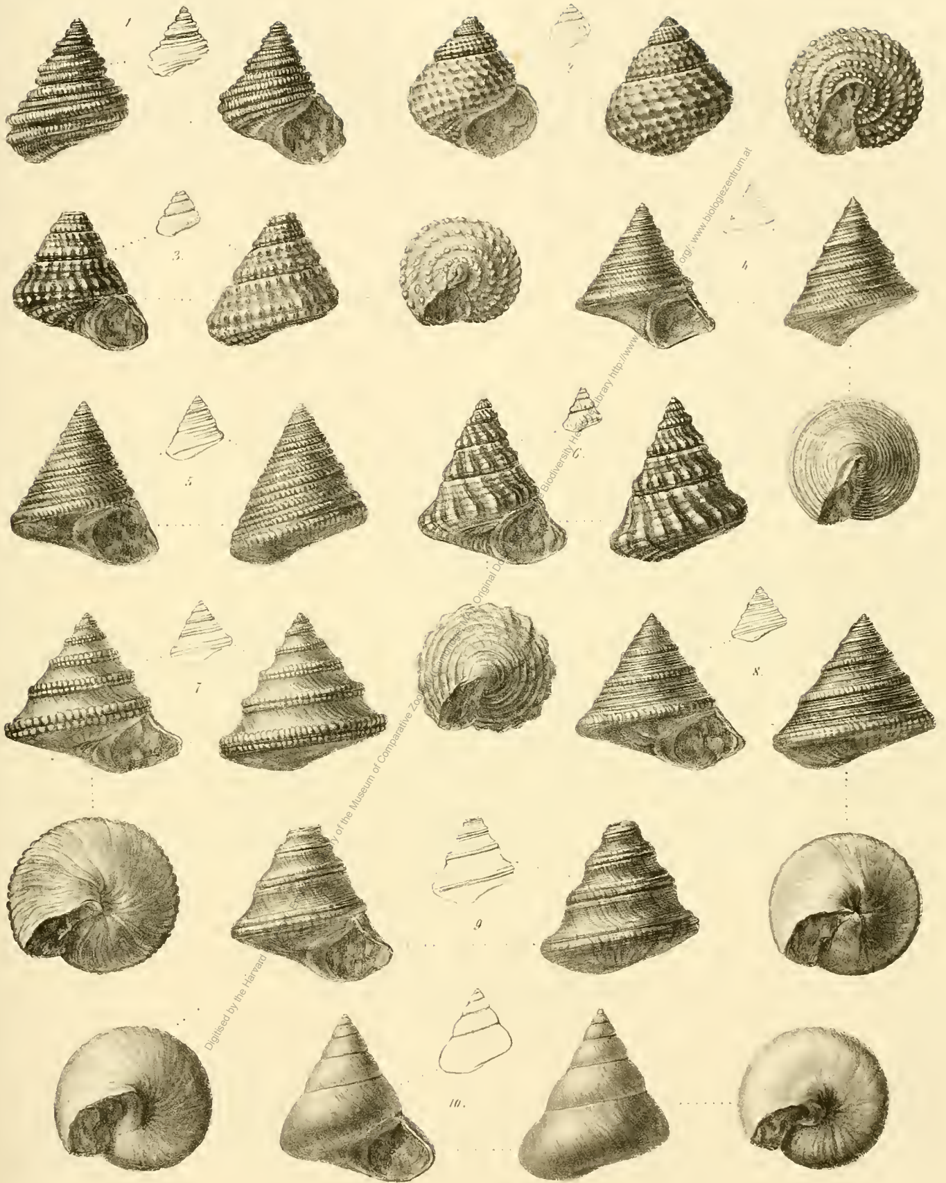
Fig. 1. Turbo Davidsoni Lbe. Fig. 2. Maoidonta granaria Hebt & Deslg. Fig. 3. Maoidonta barmata Mst. Fig. 4. Tridus Baliensis Lbe. Fig. 5. Tridus entradus Lbe. Fig. 6. Tridus Viaticensis d'Orb. Fig. 7. Tridus duplicatus Sam. Fig. 8. Tridus Smythensis Laube. Fig. 9. Tridus faustus Lbe. Fig. 10. Tridus Halesus d'Orb.
