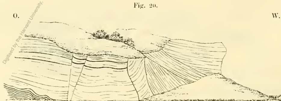
Plattige Kalkbänke mit Verwerfungen.
