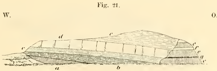
a Blauer Tegel mit kohligem Lignit. — b Travertin. — c Kalkplatten und Mergel. — d Kalkbank. — e Blauer Tegel. — f. Kalkbänke mit Melanopsis und Bithunia . — g Lignit mit Planorbis und Lymnaeus .
