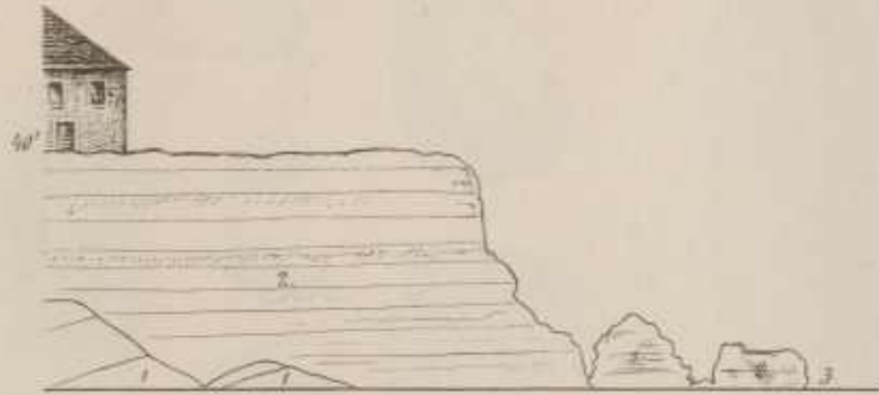
Quaternäre Muschelbänke bei Gallipoli.
