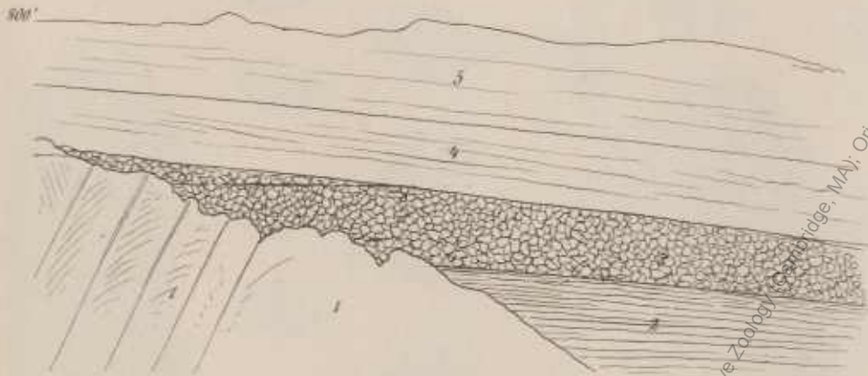
Tertiärbildungen 12 Meilen nordöstlich von Renkiöi.
