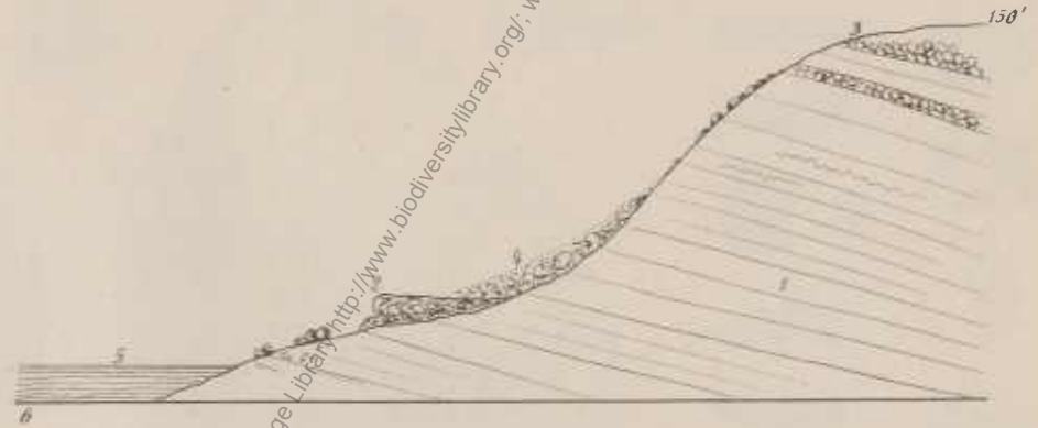
Quaternäre Muschelbänke bei Tschenek-Kalessi.
