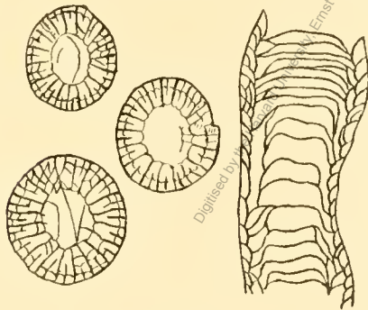
Cyathophyllum concinnum Lonsd. sp. Untercarbon. Ost von Bashsugun, Altum Artush. Quer- und Längsschliff. 3:2.
