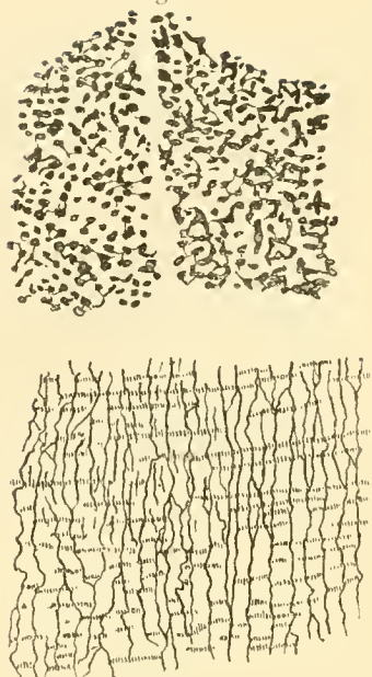
Clathrodictyon Montis Casii Frech. Ob. Mitteldevon. Mittl. Kuen-Lün. 9: 2.
