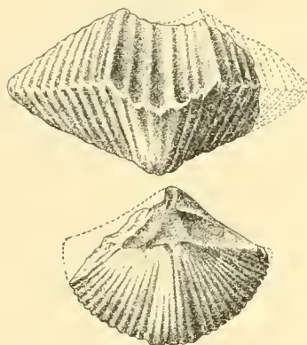
Spirifer aperturatus Schl. var. latistriata Frech. Blankenheim. Crinoidenschicht. Coll. Frech. 1:1 und 3:2.
