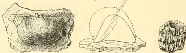
Productus tibeticus Frech. Unterdyadischer Brachiopodenkalk vom Fl. Gussass. Links kleine Klappe mit Schlossfortsatz (von innen), rechte Oberflächensculptur, vergr.
