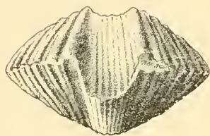
Spirifer aperturatus Schl. Original exemplar Schlotheim's, Mittl. Mitteldevon. Gegend von Köln. Mus. f. Naturkunde, Berlin. 1:1.
