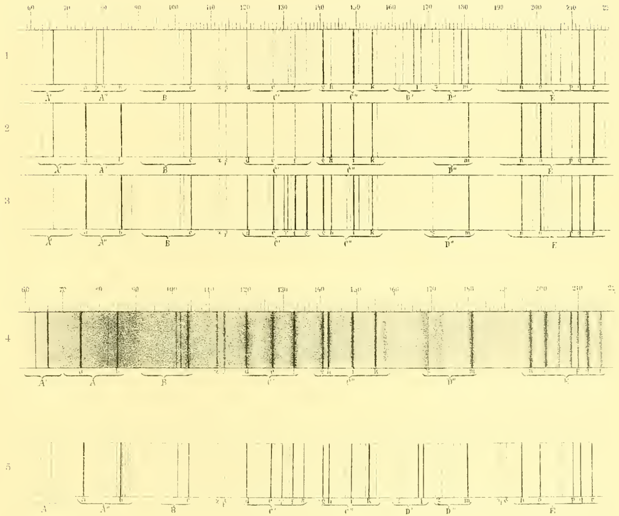
1. Brom bei stärkster Verdünnung. — 2. Bei Druck von über 10 mm. — 3. Bei etwas grösserem Drucke. — 4. Starker Dampfdruck bei 50° C. — 5. Vollständiges Spectrum des Brom nach Ciamician.
