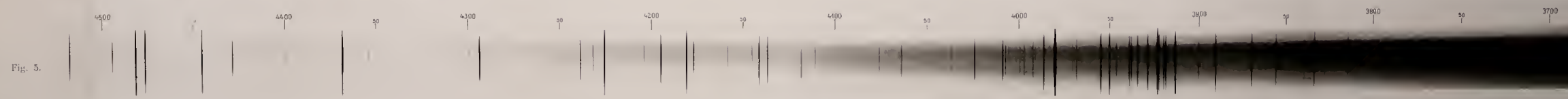
Fig. 3. Gelber bis grüner Bezirk; Druck circa 45 mm. Linien-spectrum, gemischt mit Bandenspectrum (2. Ordnung)
