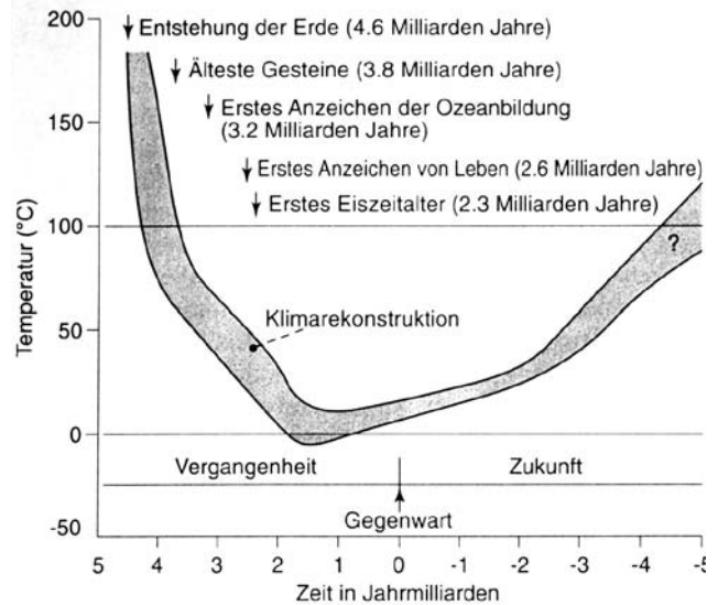
Abb. 2: Mutmaßlicher Verlauf des bodennahen Temperaturbandes in der irdischen Atmosphäre in Vergangenheit, Gegenwart und Zukunft.
