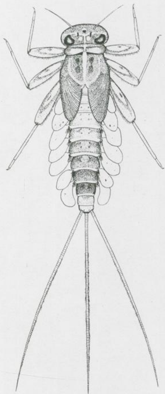
Rhithrogena semicolorata Curt., ausgewachsene Larve. Vergrößerung 6-fach.
