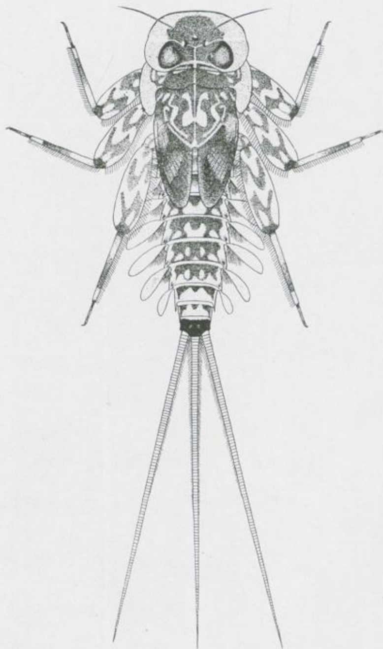
Ecydonurus venosus Fabr., ausgewachsene Larve. Zur besseren Darstellung der Kiemenbüschel sind hier die Kiemenblättchen schräg gestellt und daher in der Breite perspektivisch verkürzt. Vergrößerung 5-fach.
