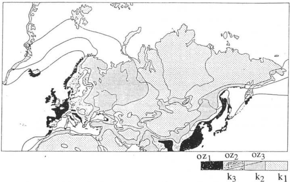
Abb. 2: Ozeanitätsstufen in Eurasien. Entwurf Jäger (JÄGER 1968)
