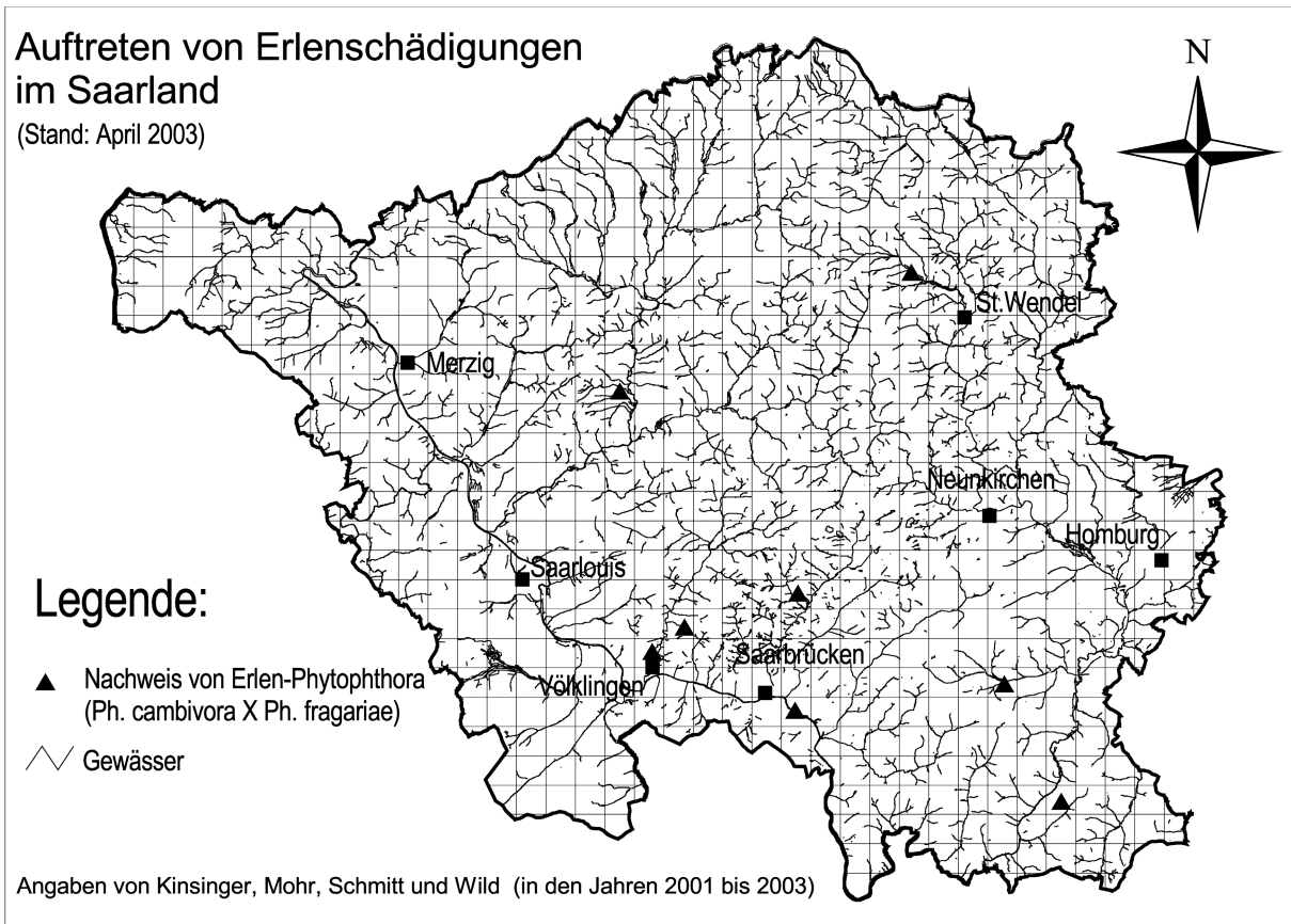
Abb. 1: Derzeitige Situation von neuartigen Erlenschädigungen im Saarland (Stand: April 2003). Kartografie: V. Wild, 2003
