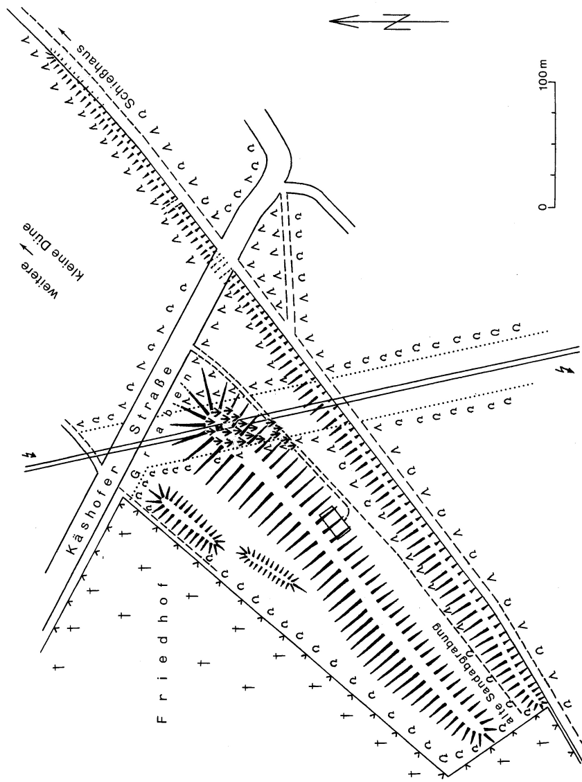
Abb. 5: Lage und Gliederung des Dünenkomplexes östlich des Homburger Friedhofs. Büschel-Signatur: Sandtrockenrasen-Gesellschaften
