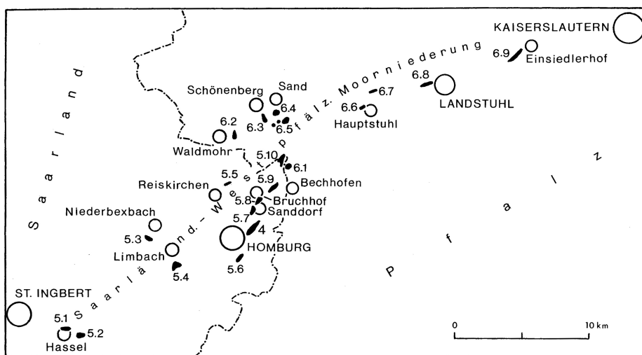
Abb. 4: Die Lage der Dünen und übrigen Flugsande an den Rändern der Saarländisch-Westpfälzischen Moorniederung. (Die schwarzen Flächen sind zur besseren Erkennbarkeit etwas vergrößert gezeichnet. Ihre Nummerierung entspricht derjenigen der betreffenden Textkapitel.)
