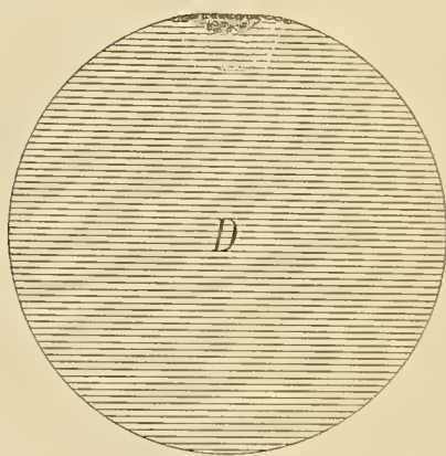
Monotremen. Uebergang der Morula ( E_3 , O_1 ) in die Blastula ( O_2 ).
