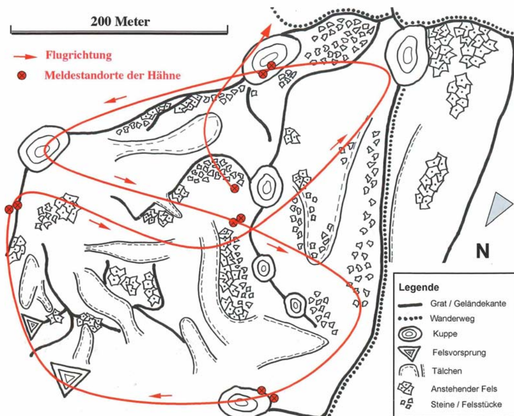
Abbildung 5: Skizze der Meldestandorte und des Verfolgungsfluges von drei territorialen Hähnen.
