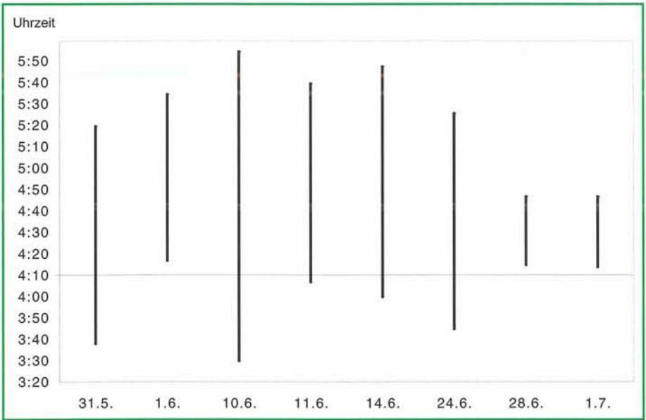
Abbildung 3: Dauer der morgendlichen Gesangsaktivität im Untersuchungszeitraum.
