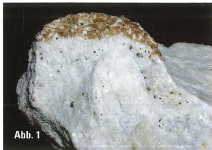
Abb. 1: Stufe, bestehend aus einem Filz von etwa 2 cm langen, weißlichen Tremolitstängeln. Randlich befindet sich eine Phlogopitschliere. Bildbreite etwa 5 cm. Sammlung und Foto H. Offenbacher, Graz.
