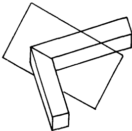
Abb. 4 Verzwillingung als möglicher Grund f.d. Bildung rechtwinkl. Nadelpyrite. Zwillingssebene (110)
