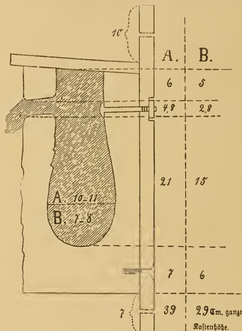
Längsschnitt mit Maßangaben.
