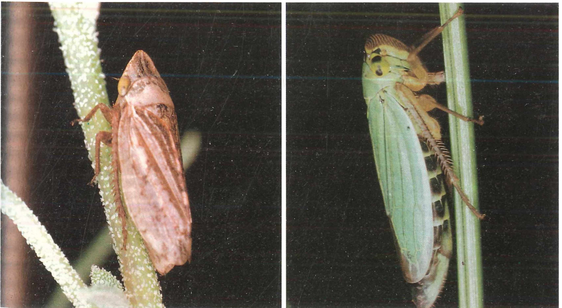
Abb. 2: (a) - Aphrodes costatus , auf beiden Inseln häufig; (b) - Cicadella viridis , auf dem Festland häufig, auf den jungen Inseln nur vereinzelt. — Fig. 2: (a) - A. costatus , abundant on both islands; (b) - C. viridis , abundant on the mainland, on the young islands rarely present.
