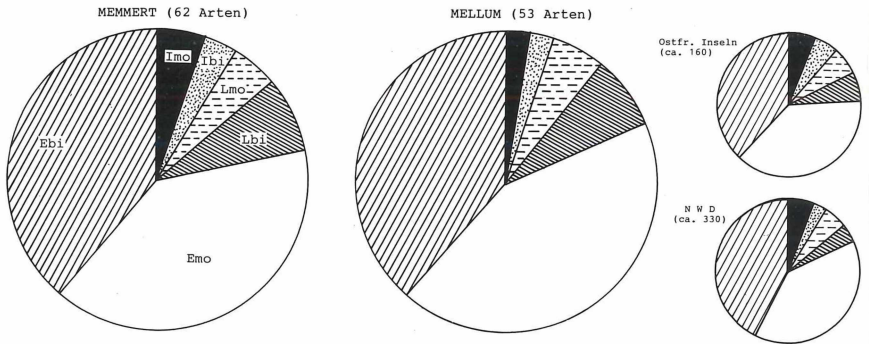
Abb. 5: Zusammensetzung der Zikadenfaunen entsprechend der Nahrungspflanzenbindungen. — Fig. 5: Species composition of Auchenorrhyncha according to their host plant preferred.
