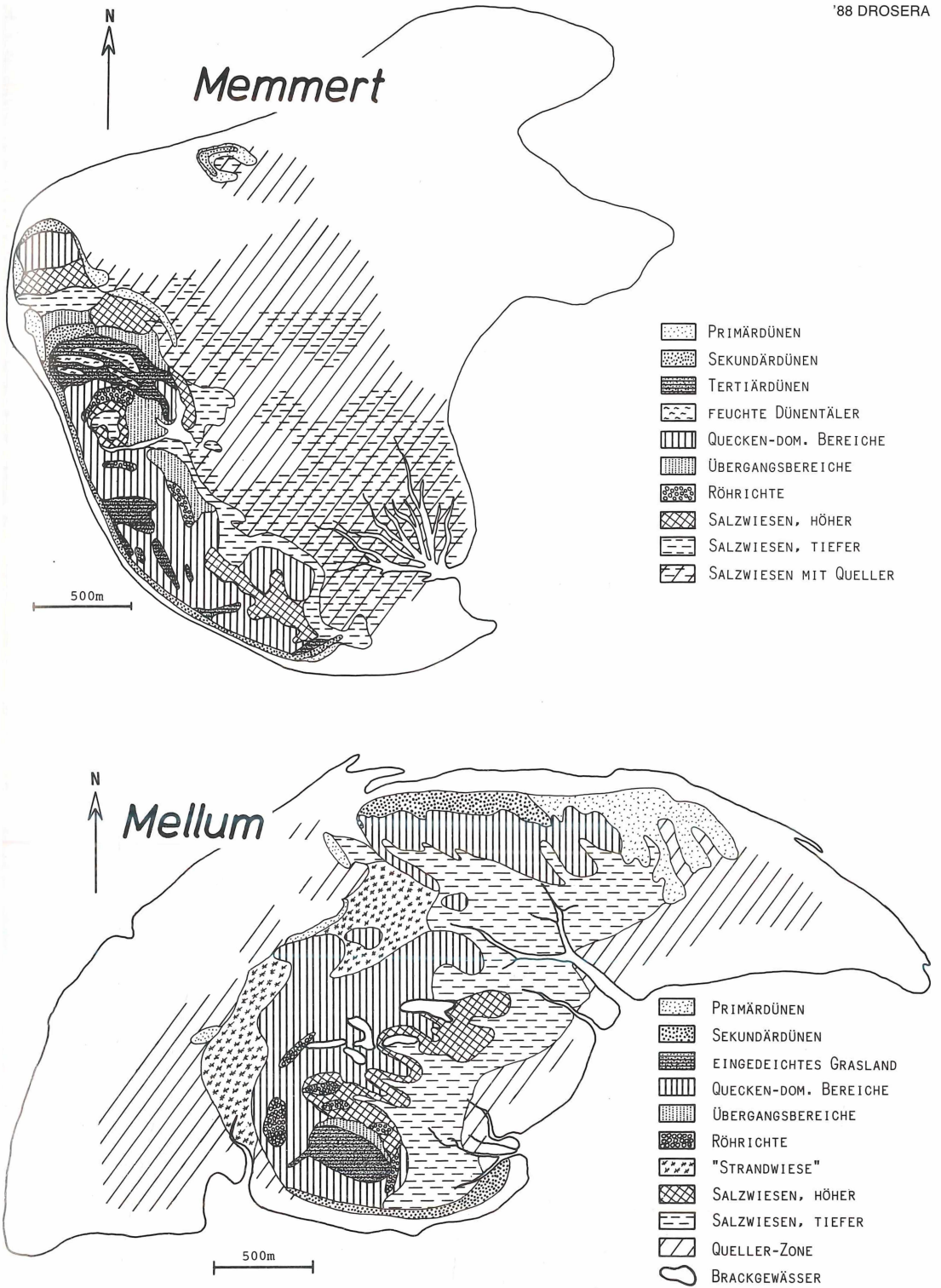
Abb. 1: Landschaftliche Gliederung von Memmert (nach RESING 1979, verändert u. ergänzt) und Mellum (nach KUHBIER 1987, verändert u. ergänzt). — Fig. 1: Outline of landscape and habitat structure of Memmert and Mellum, according to RESING 1979 and KUHBIER 1987, modified and completed.
