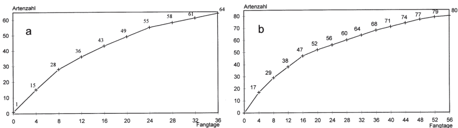
Abb. 7: Artenarealkurve für (a) Grabwespen und (b) Bienen
