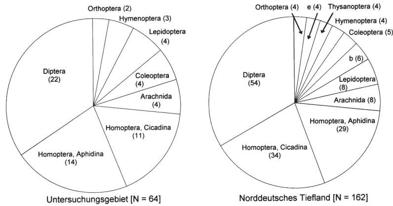
Abb. 10: Beutetierspektrum der Grabwespenarten des Untersuchungsgebietes [Zuordnung nach DOLLFUSS (1991), OEHLKE (1970), OLBERG (1959), SCHMIDT (1979, 1980, 1981, 1984)] bzw. des Norddeutschen Tieflandes [verändert nach HAESELER (1985), e = Arten mit engem Beutetierspektrum, b = Arten mit breitem Beutetierspektrum, in ( ) = Anzahl der Arten].
