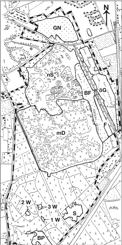
Abb. 1: Übersichtsplan „Standortübungsplatz Bümmerstede“ (gestricheltes Band = Grenze des Standortübungsplatzes, durchgezogene Linie = Grenze des jeweiligen Teilgebiets).
