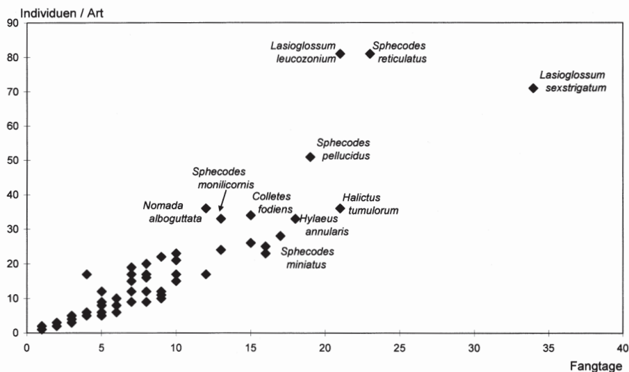
Abb. 6: Häufigkeit der einzelnen Bienenarten aufgrund der Nachweistage bzw. der nachgewiesenen Individuenzahlen (Arten mit hohen Individuen- und Tageszahlen sind namentlich aufgeführt.).
