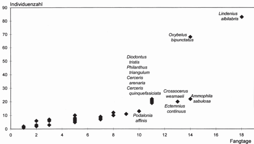
Abb. 5: Häufigkeit einzelner Grabwespenarten aufgrund der Nachweistage bzw. der nachgewiesenen Individuenzahlen (Arten mit hohen Individuen- und Tageszahlen sind namentlich aufgeführt.).
