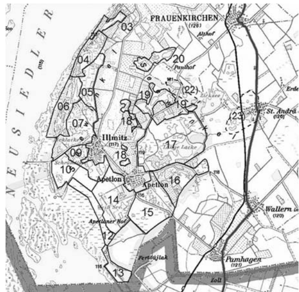
Abb. 1: Lage und Nummerierung der im Text erwähnten Teilgebiete (Managementeinheiten) des Nationalparks Neusiedler See-Seewinkel. (Bezeichnungen s. Tab. 1). Die Teilgebiete 01 („Naturzone“), 02 („Zitzmannsdorfer Wiesen“) und 21 („Hanság“) wurden im Rahmen des Zählprogramms nicht kontrolliert und liegen außerhalb des gewählten Kartenausschnitts. Die strichliert umrandeten „Teilgebiete“ 22 und 23 gehören nicht zum Nationalpark und wurden für den Zweck dieser Auswertung geschaffen. Kartengrundlage: Austrian Map – Bundesamt f. Eich- und Vermessungswesen.
