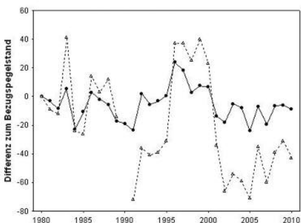
Abb. 6: Langfristige Wasserstandsentwicklung der Langen Lacke (helle Dreiecke) und an sechs weiteren Lacken (schwarze Kreise); nähere Erläuterung im Text.
