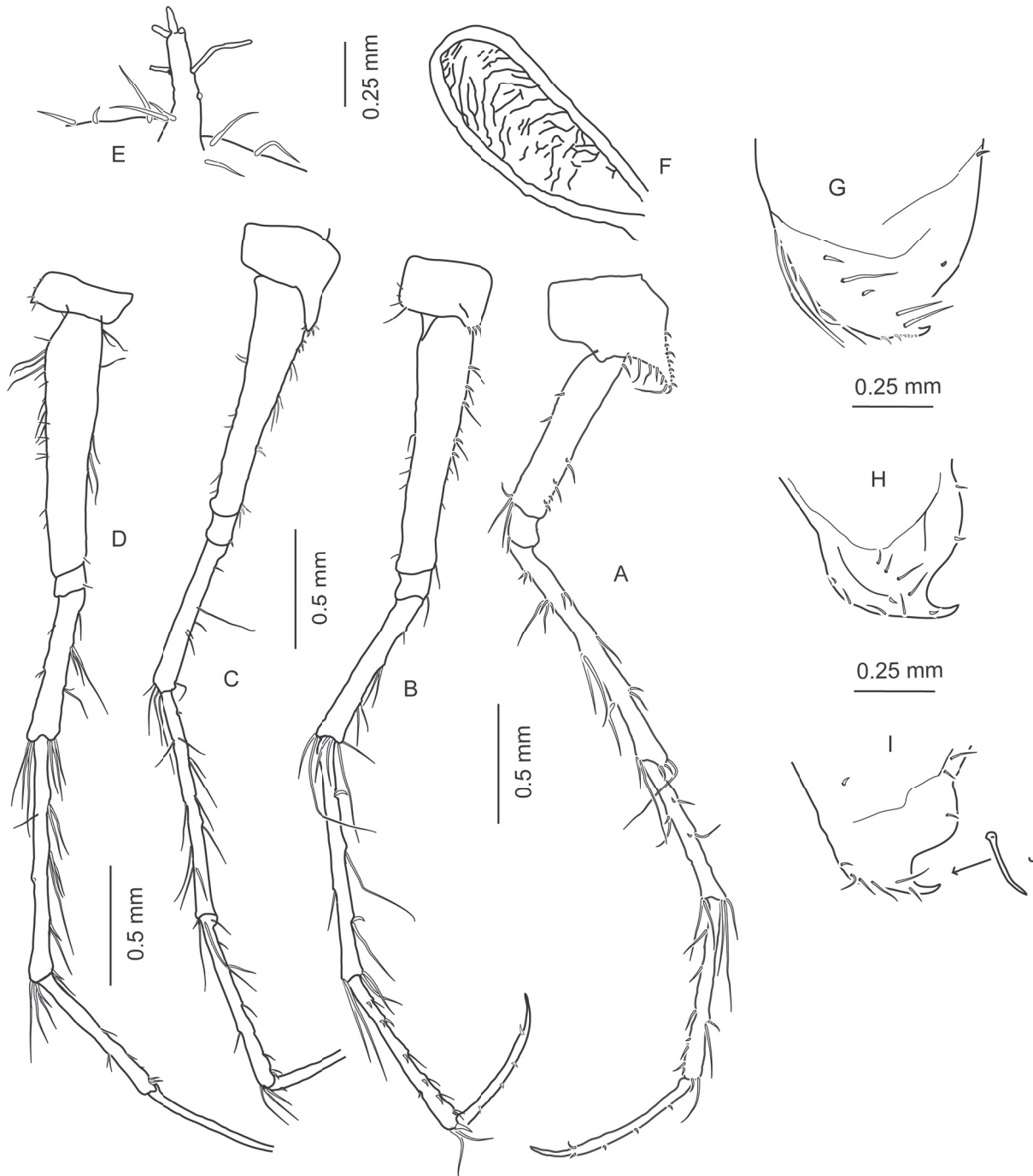
Fig. 4. Lepechinella arctica , holotype, ♀. A. Right P4. B. Right P6. C. Right P5. D. Right P7. E. Tooth of peraeon segment 6. F. Gill of P5. G. Ep1. H. Ep2. I. Ep3. J. Spine on Ep3.
