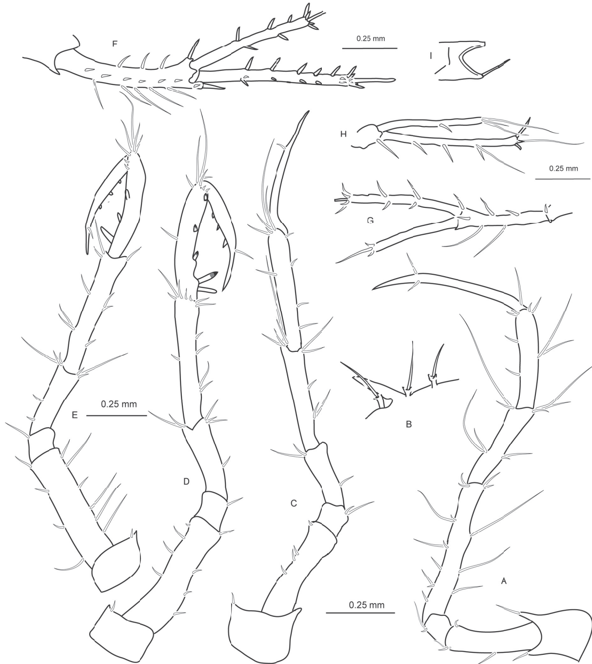
Fig. 19. Lepesubchela christinae gen. et sp. nov., holotype, immature. A. Left P4. B. Tooth of pereon segment 5. C. Left P5. D. Left P6. E. Right P7. F. Left U1. G. Right U2. H. U3. I. Telson.
