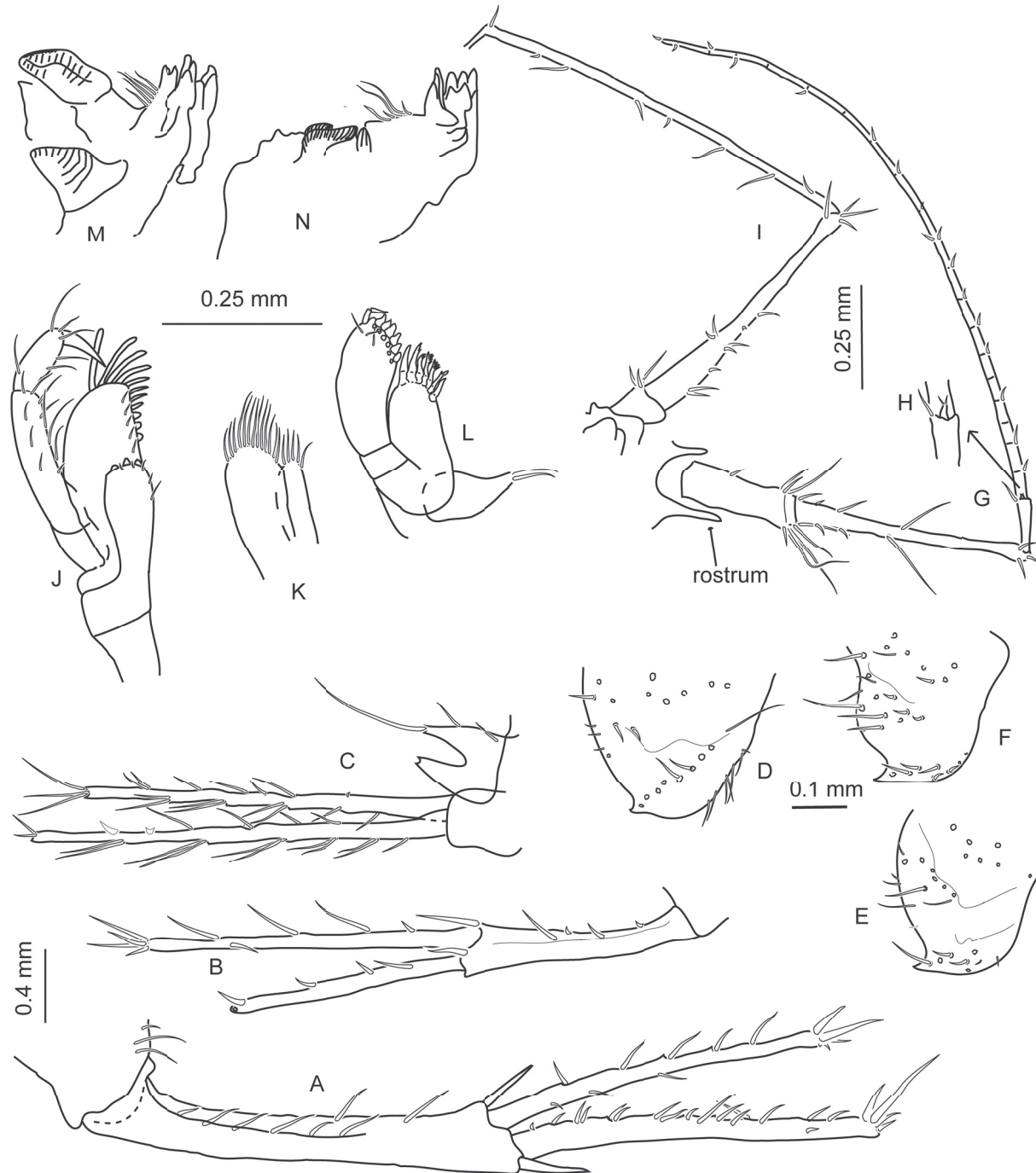
Fig. 11. Lepechinella schellenbergi Stephensen, 1944, lectotype, ♀. A. Left U1. B. Right U2. C. Right U3 and telson. D. Right Ep1. E. Right Ep2. F. Right Ep3. G. Female A1. H. Accessory flagellum. I. Female A2. J. Left Mxp. K. Left Mx2. L. Left Mx1. M–N. Left and right mandible.
