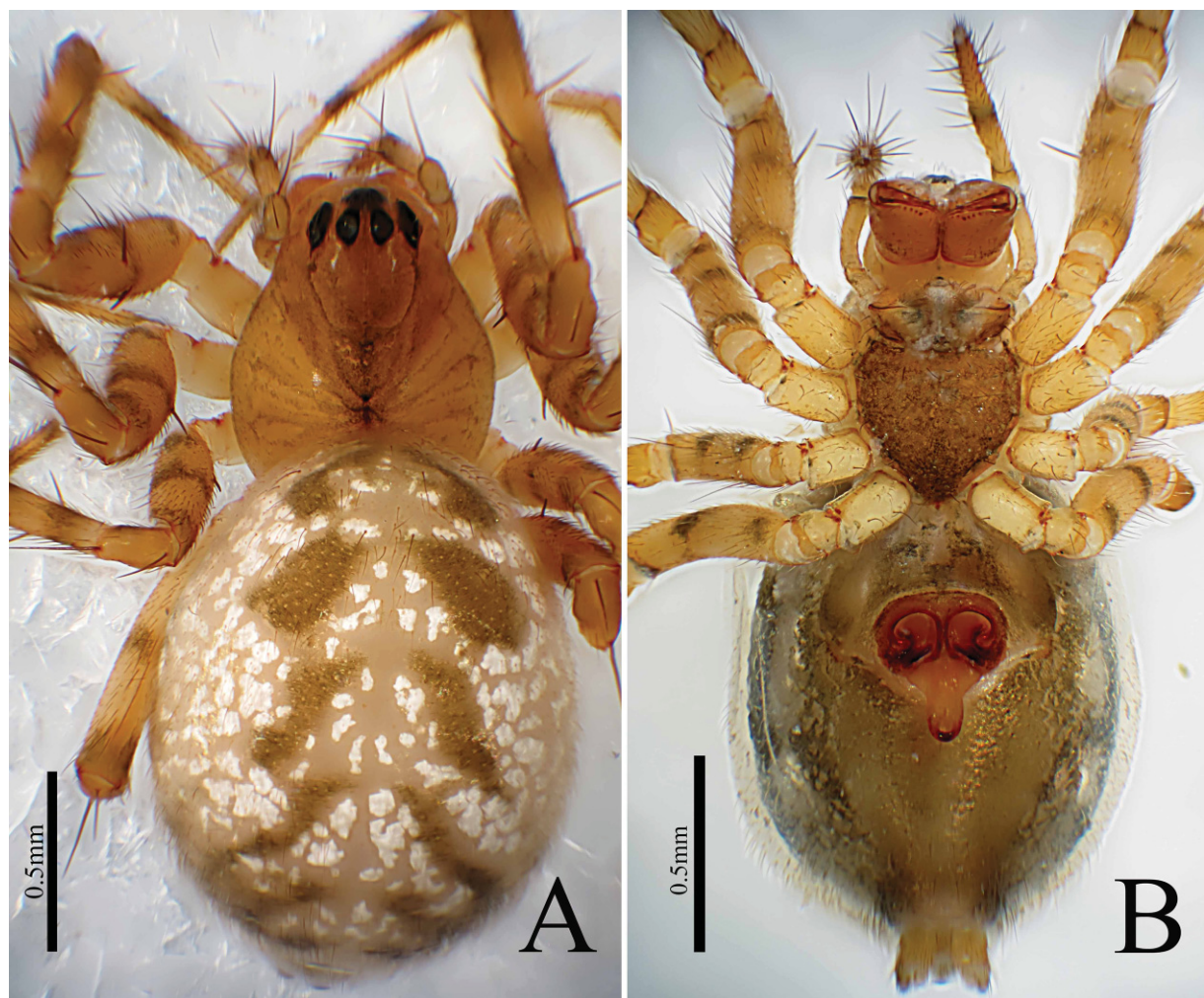
Fig. 23. Acroterius inversus gen. et sp. nov., ♀, holotype (HNU-CGY115). A. Habitus, dorsal view. B. Habitus, ventral view.
