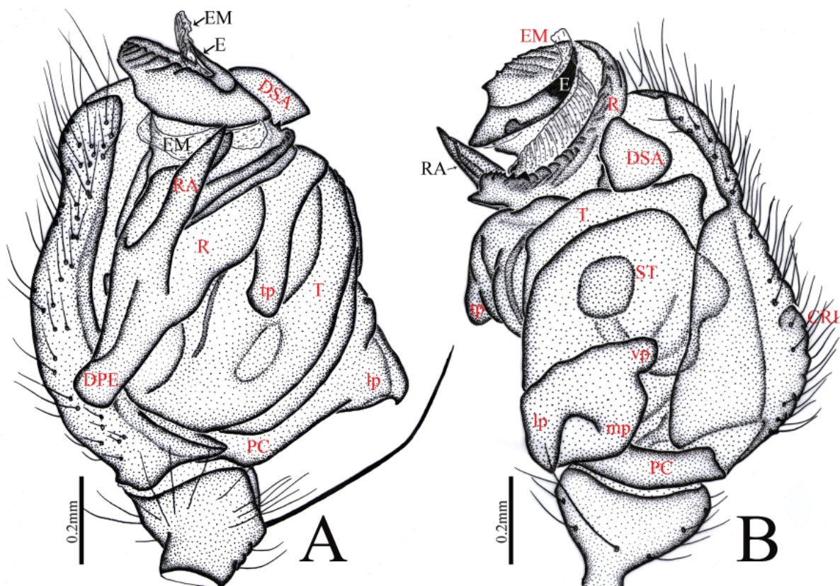
Fig. 16. Acroterius circinatus gen. et sp. nov., ♂, holotype (HNU-CGY137), palpus. A. Prolateral view. B. Retrolateral view.
