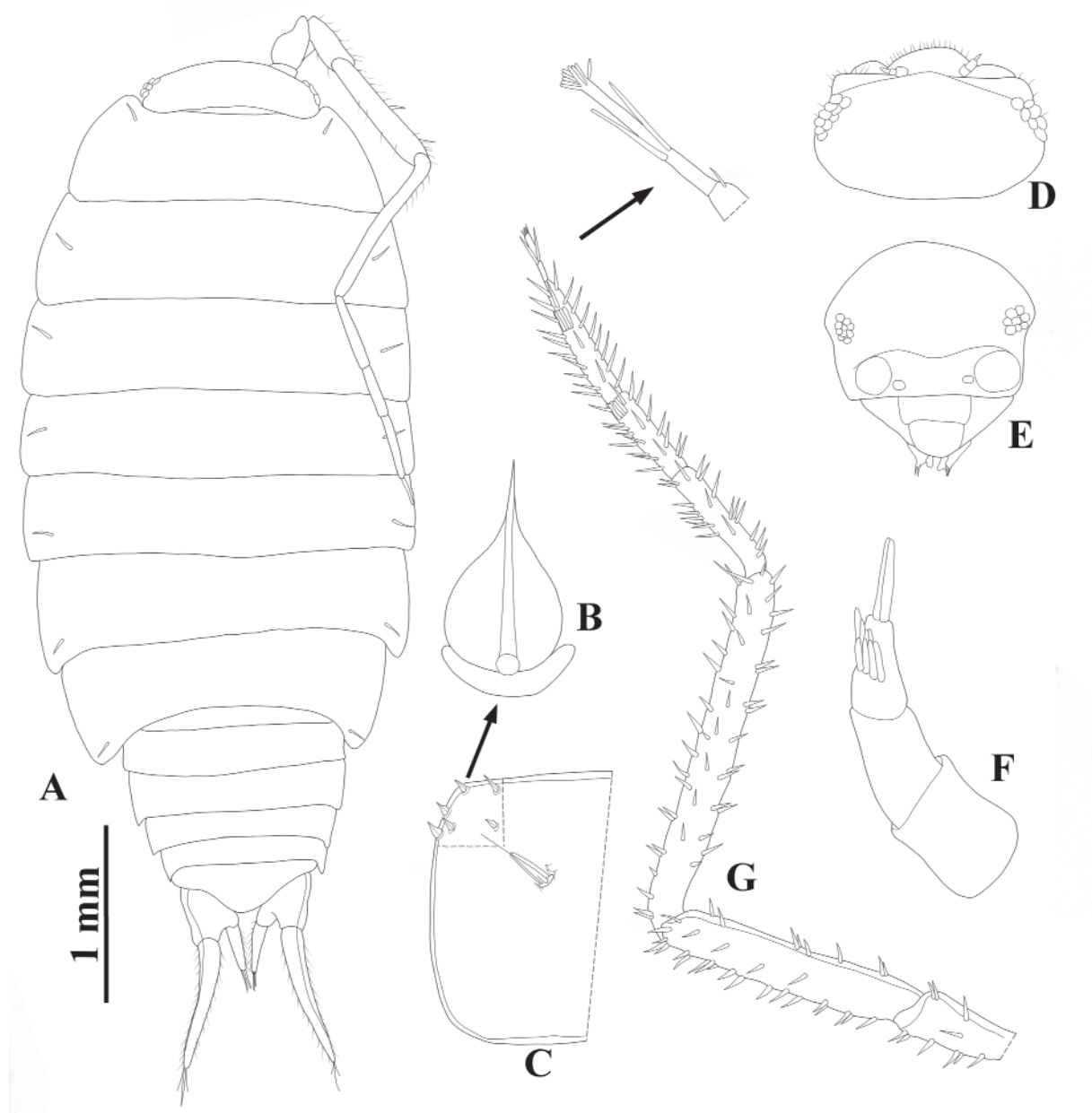
Fig. 15. Halophiloscia trichoniscoides (Vandel, 1973) comb. nov., ♀ (MZUF 9607). A. Habitus, dorsal view. B. Dorsal scale-seta. C. Epimera 4 with noduli laterales. D. Cephalon, dorsal view. E. Cephalon, frontal view. F. Antennula. G. Antenna.
