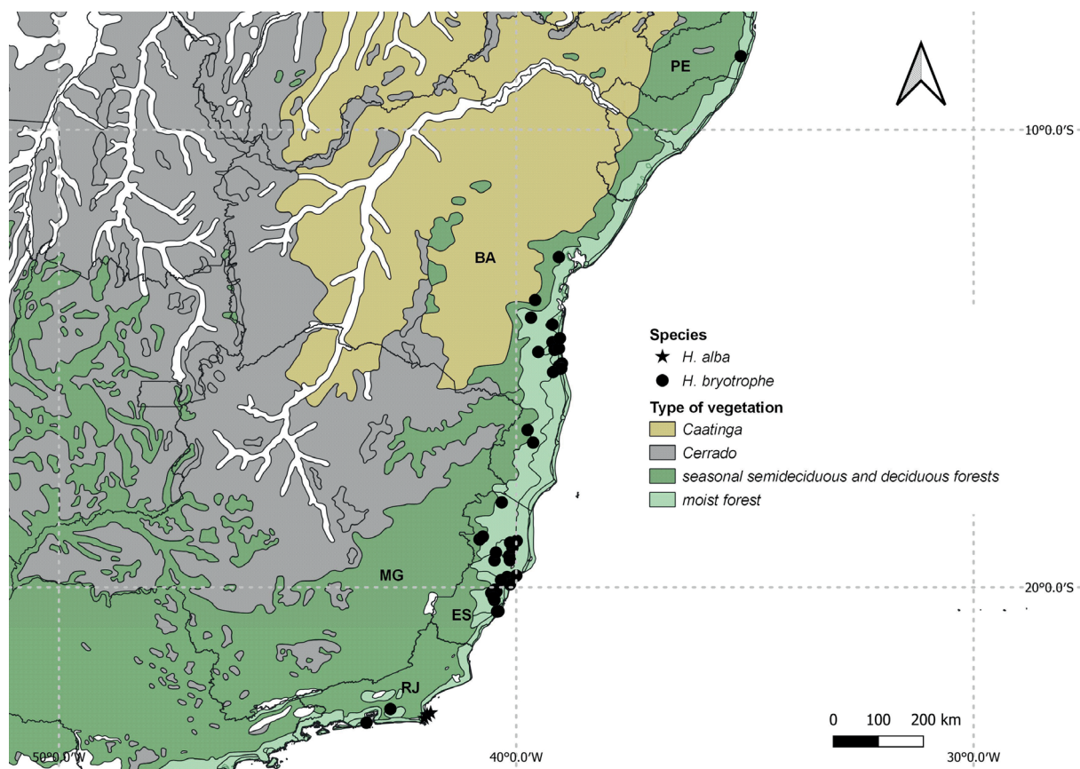
Fig. 1. Geographical distribution of Hornschuchia alba (A.St.-Hil.) R.E.Fr. and H. bryotrophe Nees. Abbreviations: BA = Bahia; ES = Espírito Santo; MG = Minas Gerais; PE = Pernambuco; RJ = Rio de Janeiro.
