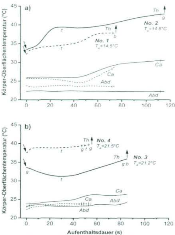
Abb. 3: Thermografisch gemessene Körper-Oberflächentemperaturen von Wasser sammelnden Honigbienen ( Apis mellifera carnica ) von Caput (Ca) Thorax (Th) und Abdomen (Abd). (a) bei niedriger und (b) bei mittelhoher Umgebungstemperatur. T_a = Umgebungstemperatur; t = trinkt, g = geht, b = bewegt sich hin und her (nach SCHMARANZER 2000).
