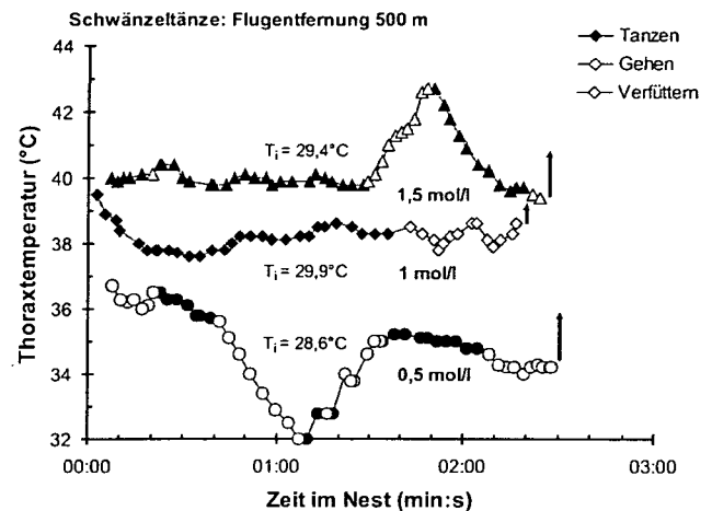
Abb. 5: Thermoregulation bei der Kommunikation im Bientanz bei verschiedener Konzentration der gesammelten Zuckerlösung. T_l = Lufttemperatur neben den Tänzerinnen (nach STABENTHEINER et al. 1995).
