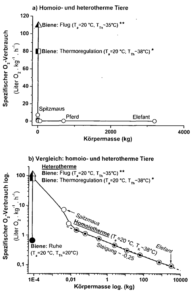
Abb. 9: Kosten der Endothermie thermoregulierender Honigbienen im Vergleich zu homoiothermen Tieren verschiedener Masse bei einer Umgebungstemperatur ( T_a ) von 20 °C. T_K = Körpertemperatur, T_{Th} = Thoraxtemperatur. (* nach Stabentheiner et al. 2003; ** nach Roberts & Harrison 1999; Homoiotherme nach Schmidt-Nielsen 1999).
