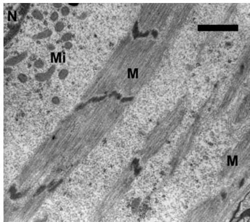
Abb. 2: Die Ventile von P. americana sind sehr plasmareich und enthalten nur wenige Myofibrillen und Mitochondrien. Balken = 1 \mu\text{m} . M – Myofibrillen, Mi – Mitochondrien, N – Nucleus.
