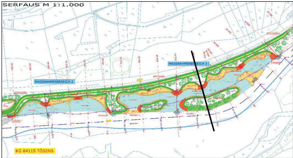
Abb. 5: Plan für die Revitalisierung Serfaus (Ausschnitt). Der schwarze Strich markiert den baulichen Fortschritt im ersten Jahr. Wasserführende Seitenarme (hellblau), Uferbefestigungen (rot), Bremsflächen (ocker), Hauptgerinne neben der Revitalisierung (Fließrichtung nach rechts) (weiß). Quelle: Büro Wasser&Umwelt im Auftrag der Abt. Umweltschutz, Amt d. Tiroler Landesregierung.
