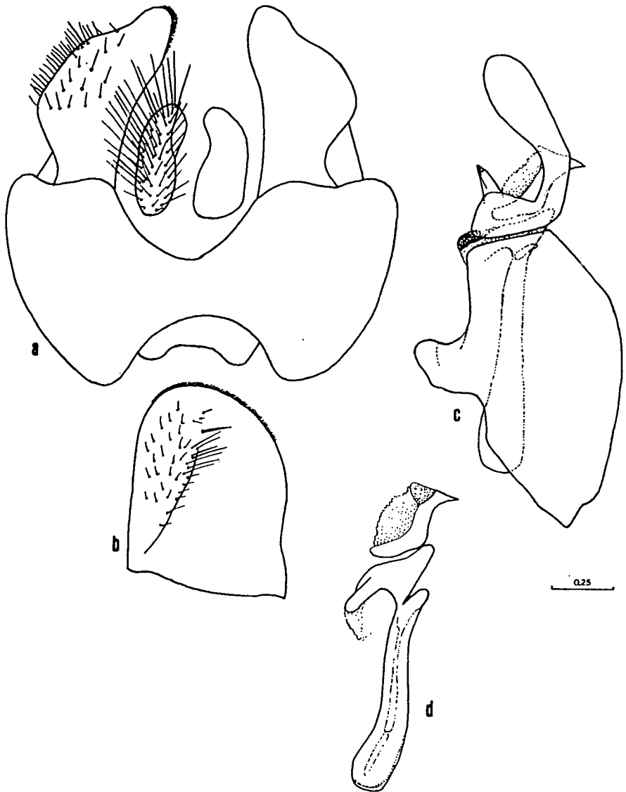
Abb.2: C. griseifacies sp. nov. (Paratypus: Serbien, Fruška gora) ♂ Genitale: a) Epanthrium, dorsal; b) Surstylus rechts, lateral; c) Hypandrium, lateral, von rechts; d) Aedoeagus und akzessorische Strukturen. - Maße in mm.
