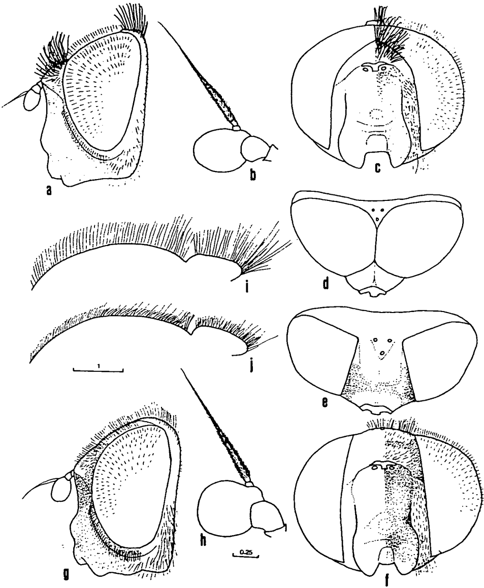
Abb.1: C. griseifacies sp. nov. (Paratypen: Serbien, Fruška gora). - a-d ♂: a) Kopf, lateral; b) Fühler, von innen; c) Kopf, frontal; d) Kopf, dorsal; - e-h ♀: e) Kopf, dorsal; f) Kopf, frontal; g) Kopf, lateral; h) Fühler, von innen; - i) Mesonotum, lateral, ♂; - j) Mesonotum, lateral, ♀. - Maße in mm.
